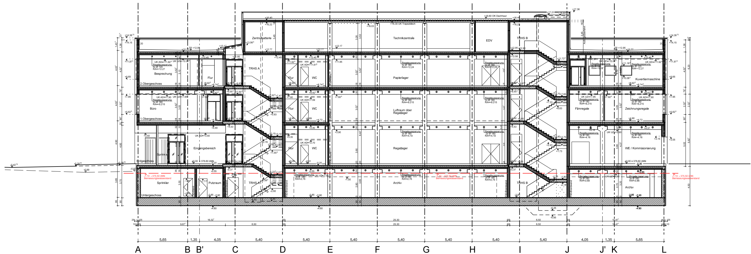
Schnitt A-A
