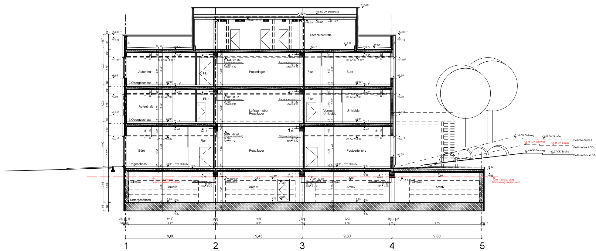
Schnitt B-B
