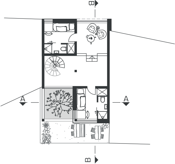
1 OG | M1:200
