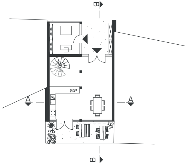
EG | M1:200
