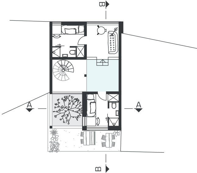
2 OG | M1:200
