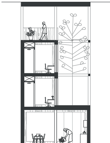
Schnitt A-A | M 1 : 200
