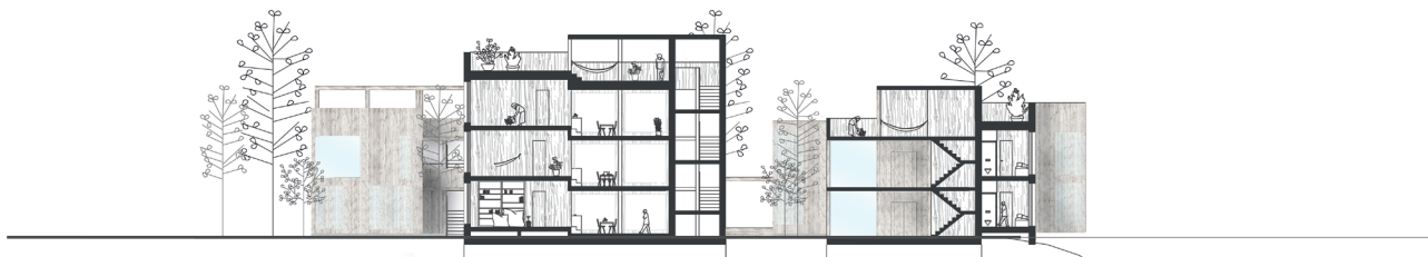
Schnitt A-A | M 1:500
