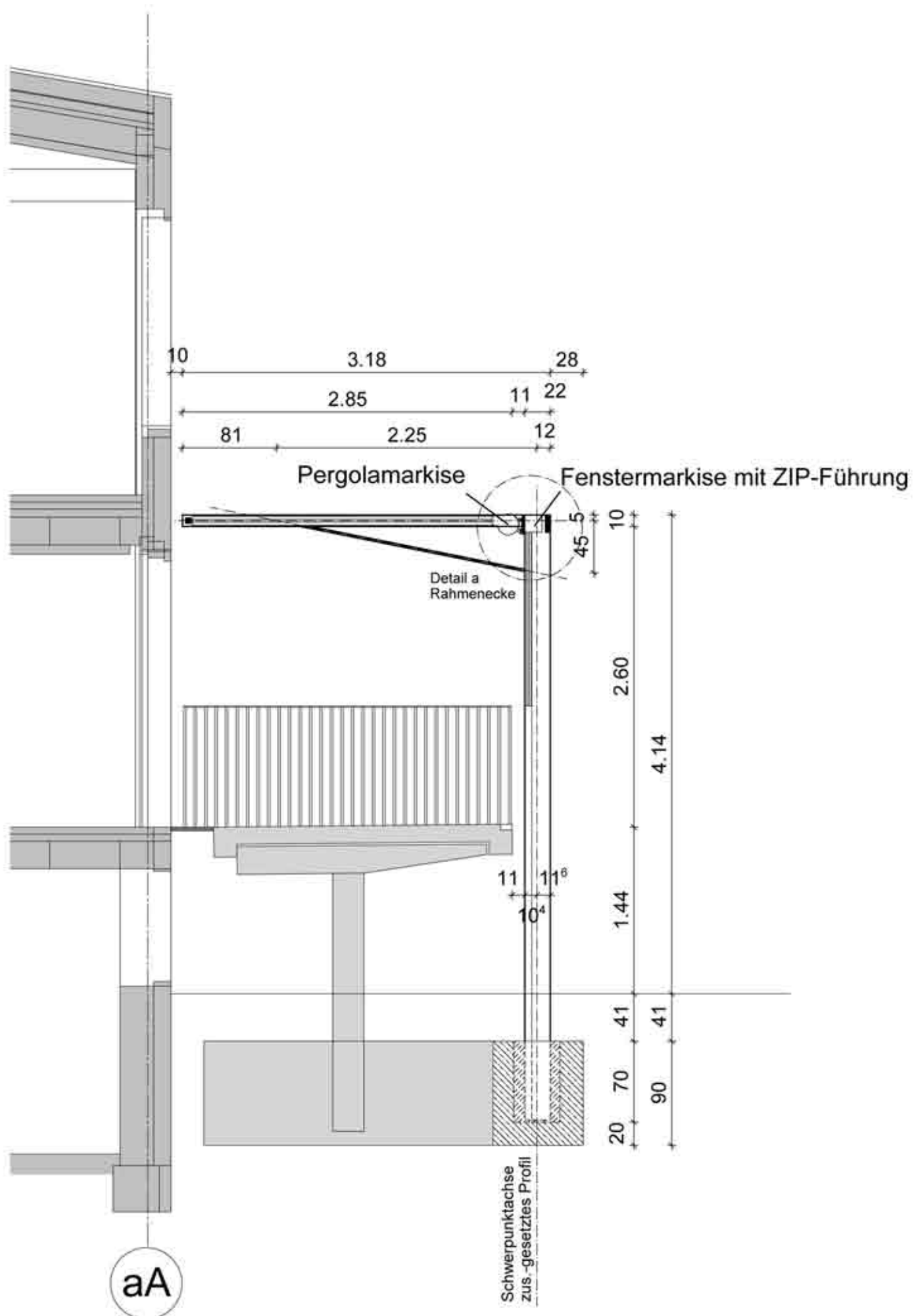
Schnitt A
