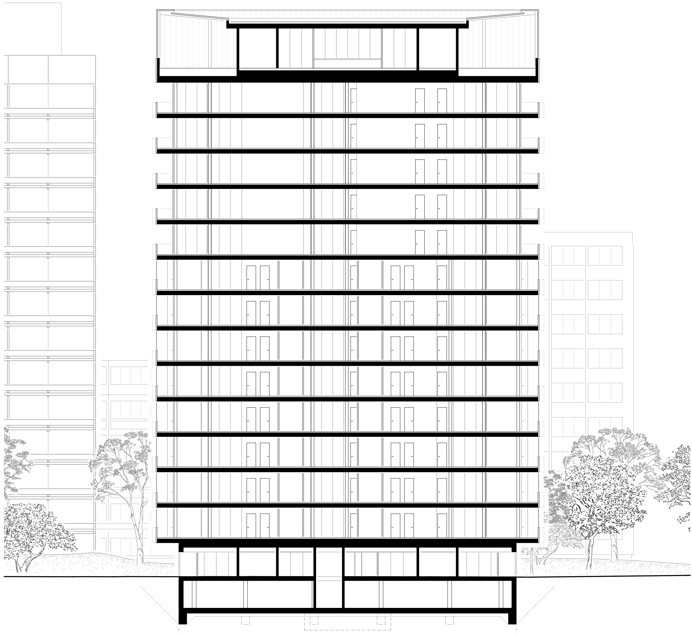
Längsschnitt
