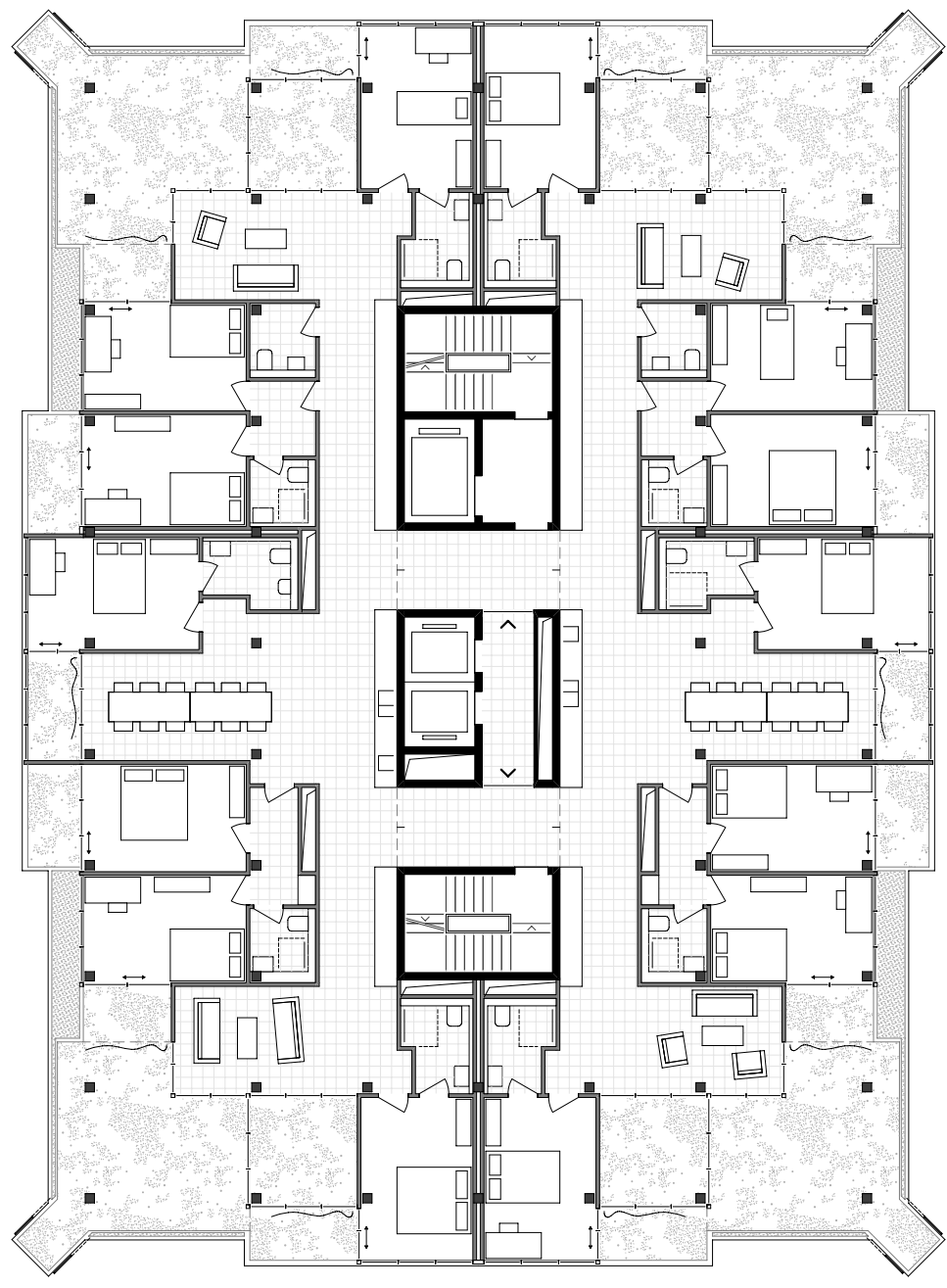
Regelgeschoss Wohngemeinschaften
