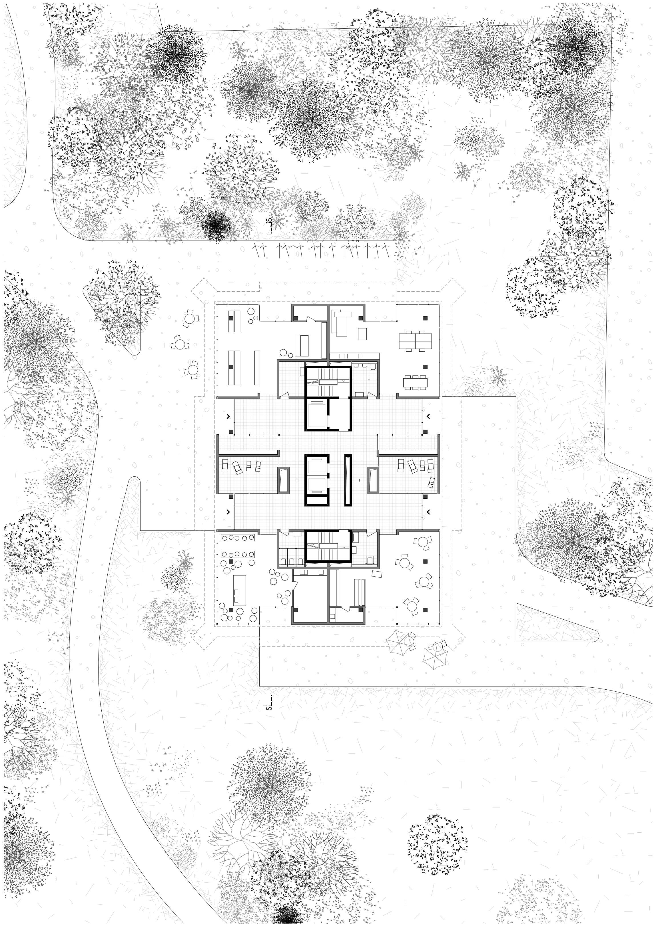
Erdgeschoss
