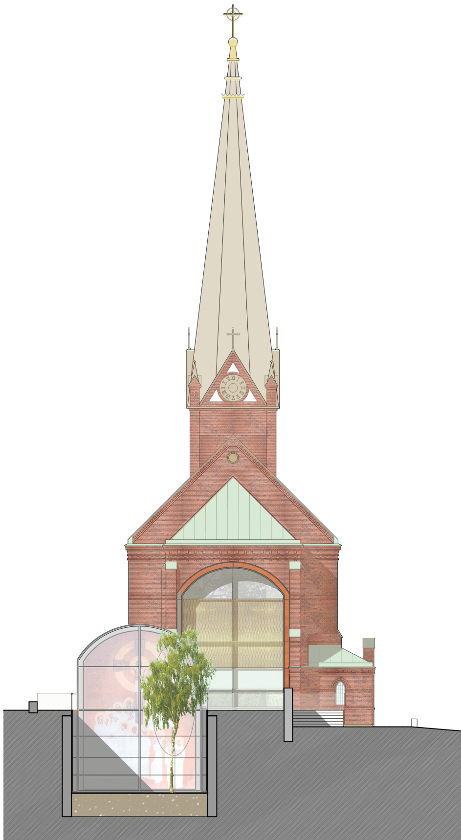
Vertikalschnitt Gedenk- und Lernort mit Ansicht Apsis 1:200
