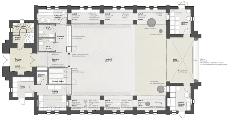
Grundriss Hauptebene
