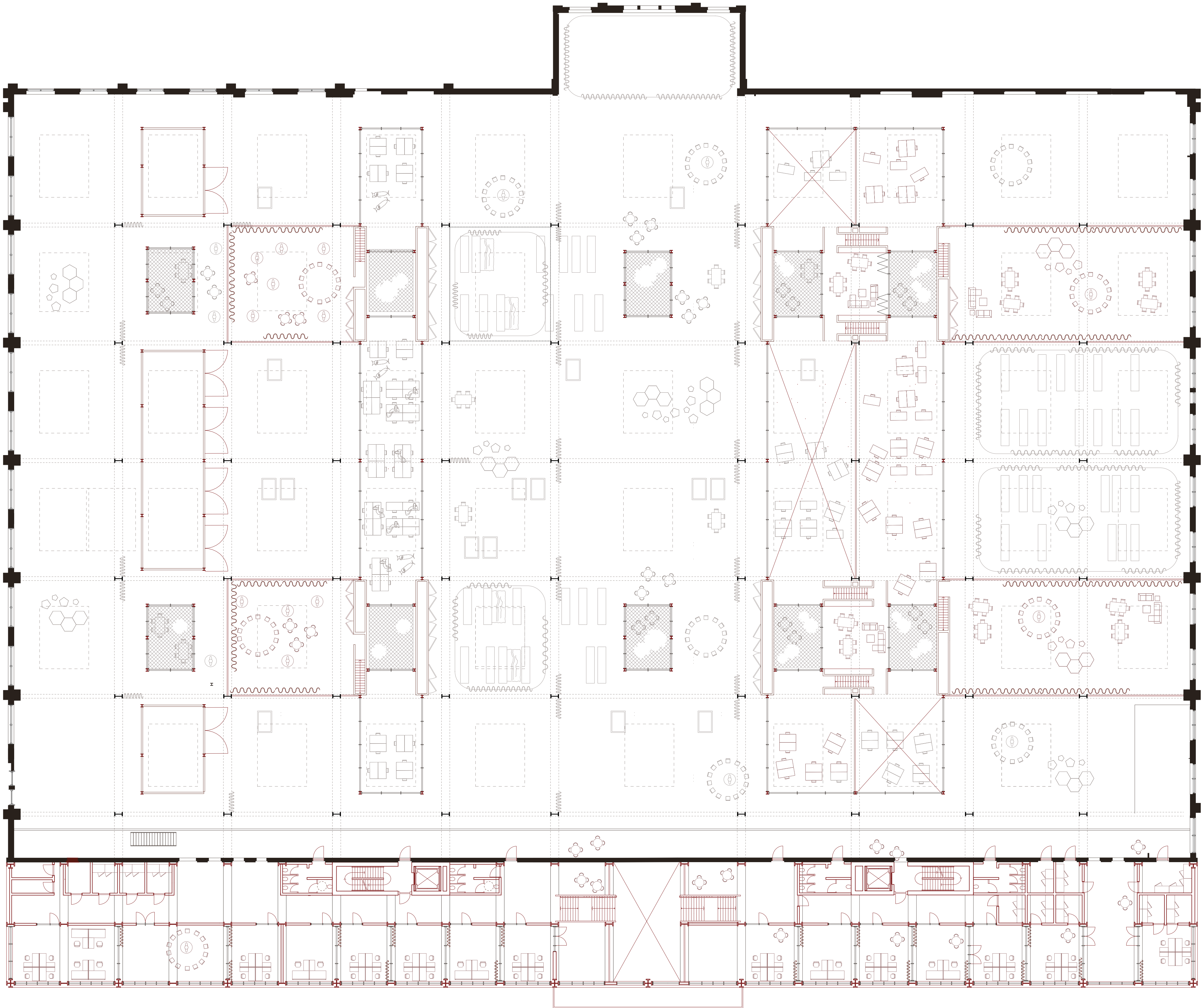
GRUNDRISS 1. OBERGESCHOSS Halle Q M 1:200
