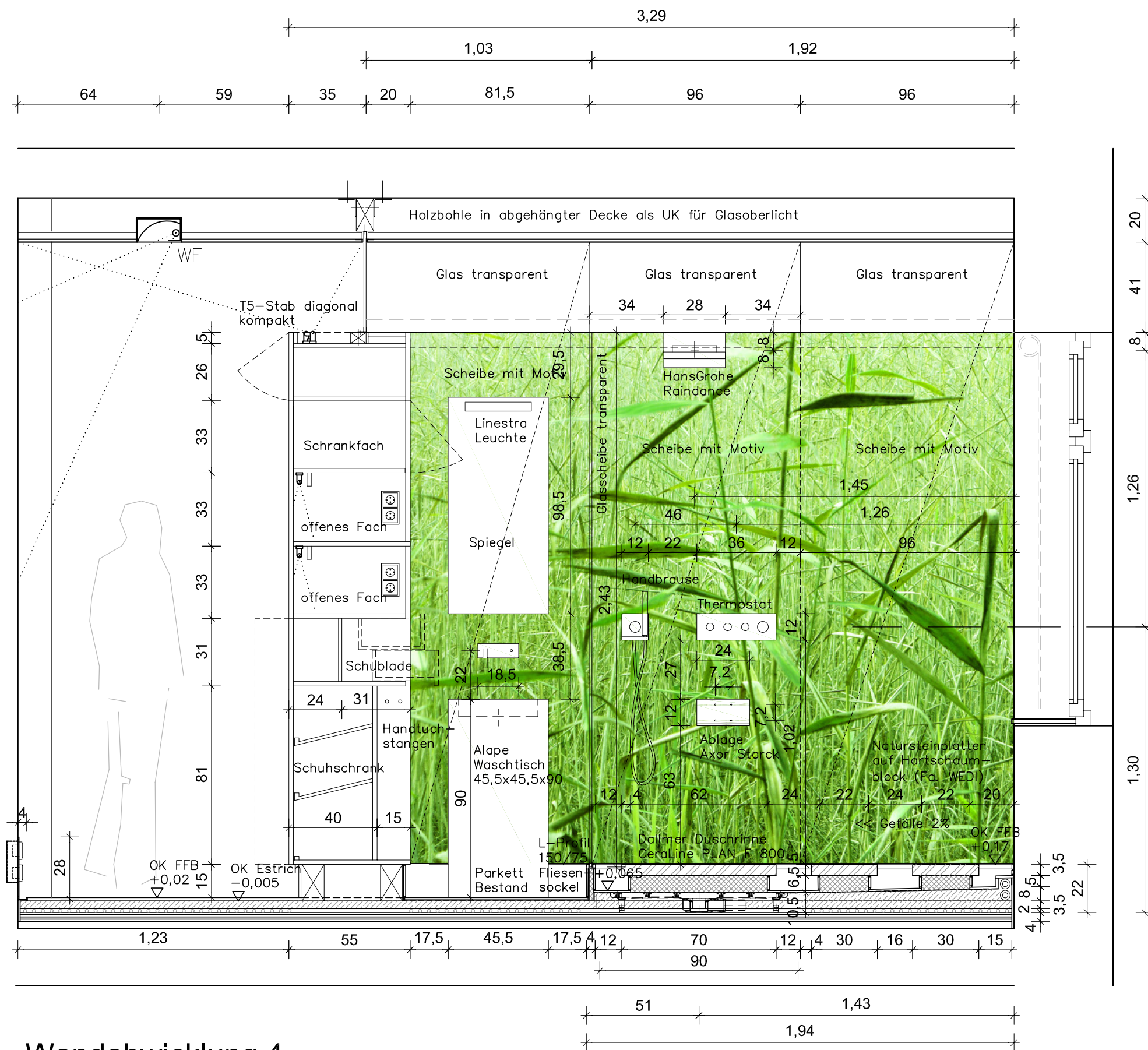
Wandabwicklung 4
