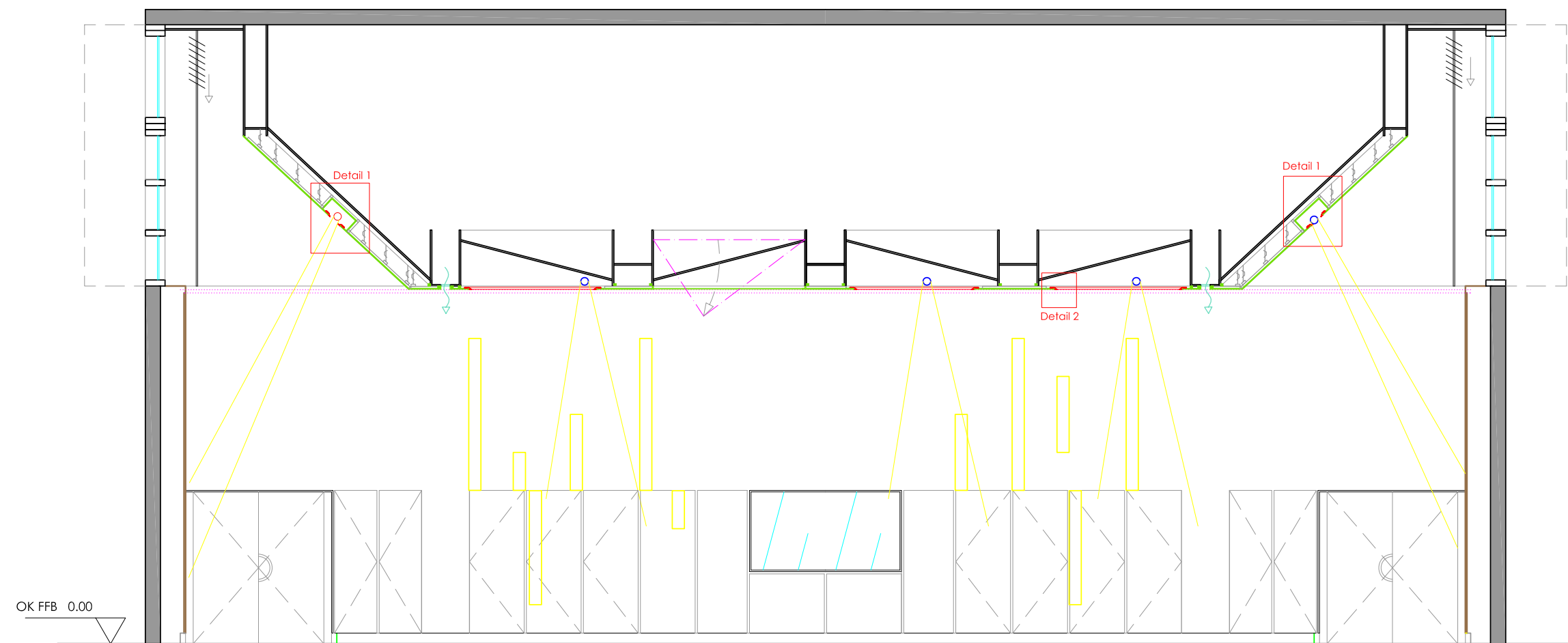
SCHNITT A-A
