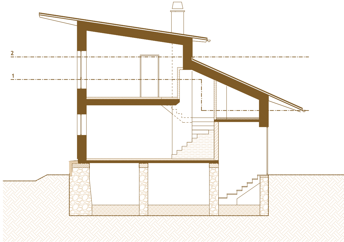
Schnitt A-A
