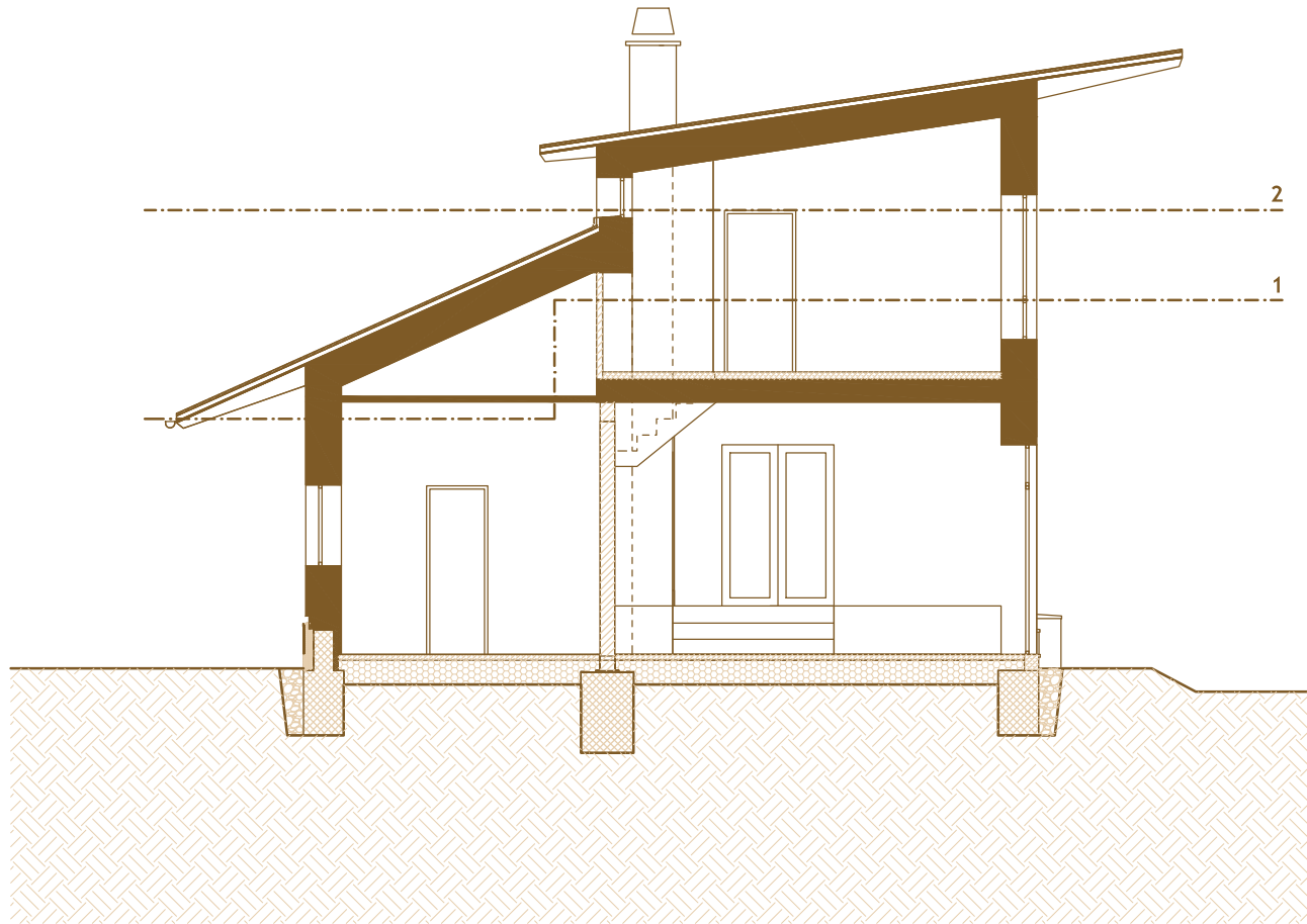
Schnitt C—C
