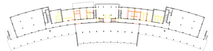
Struktur Erdgeschoss
