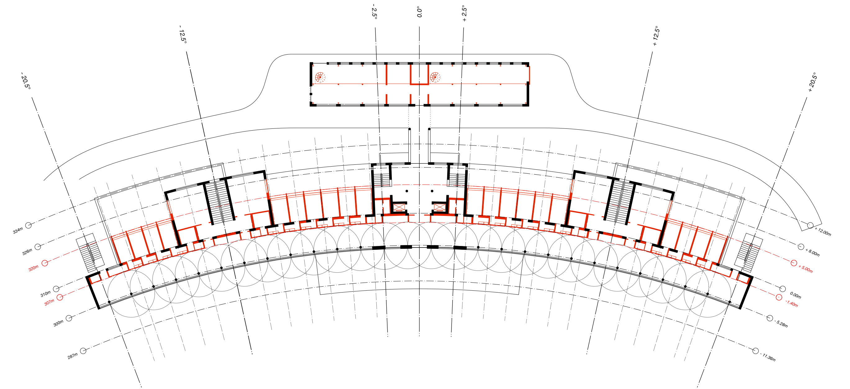
Struktur Obergeschoss
