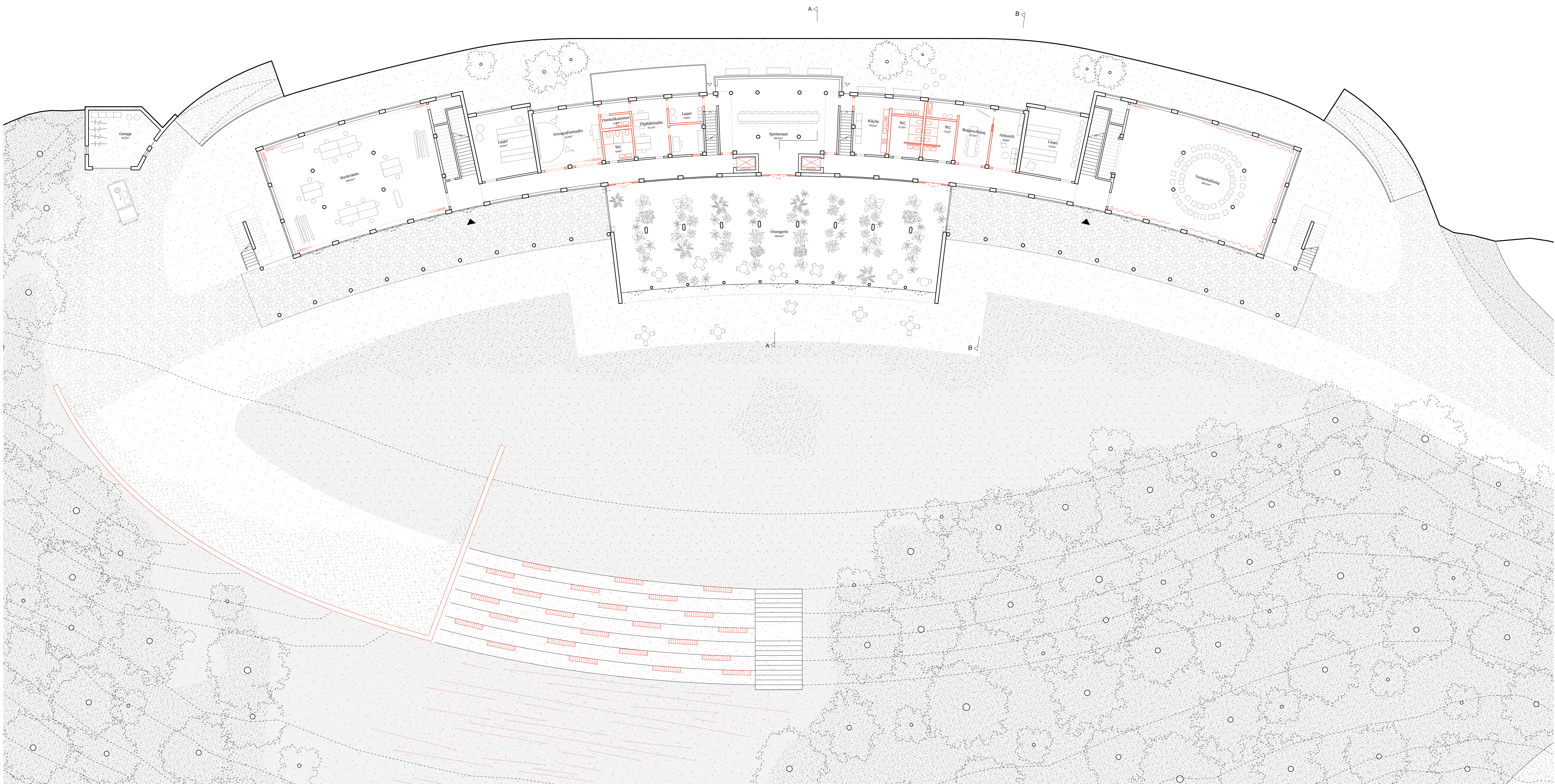
Grundriss Erdgeschoss 1:200
