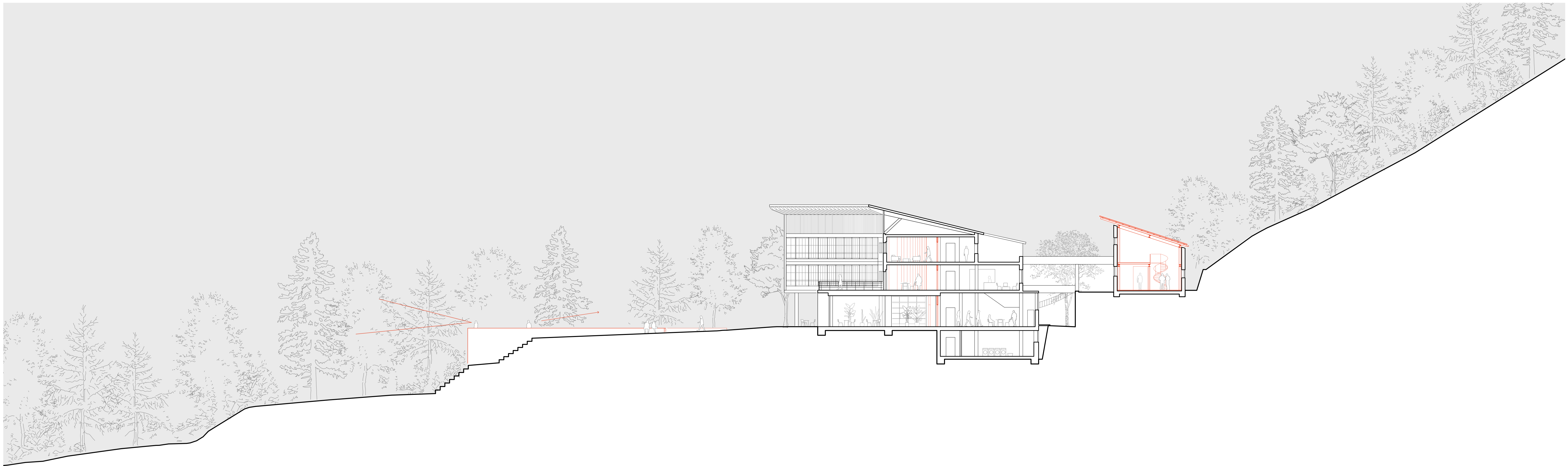
Schnitt AA + Schnitt BB 1:200
