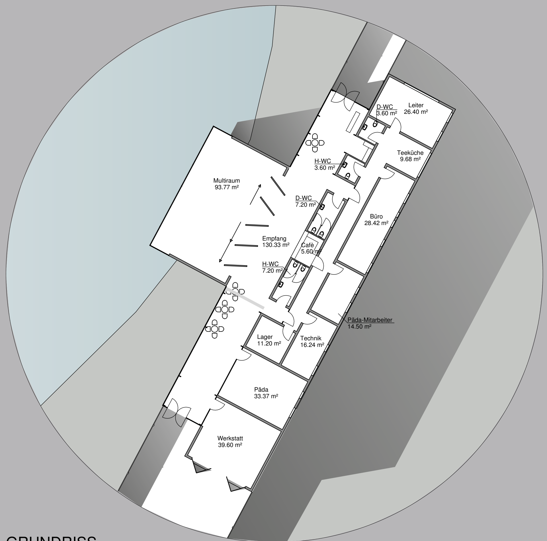
GRUNDRISS
