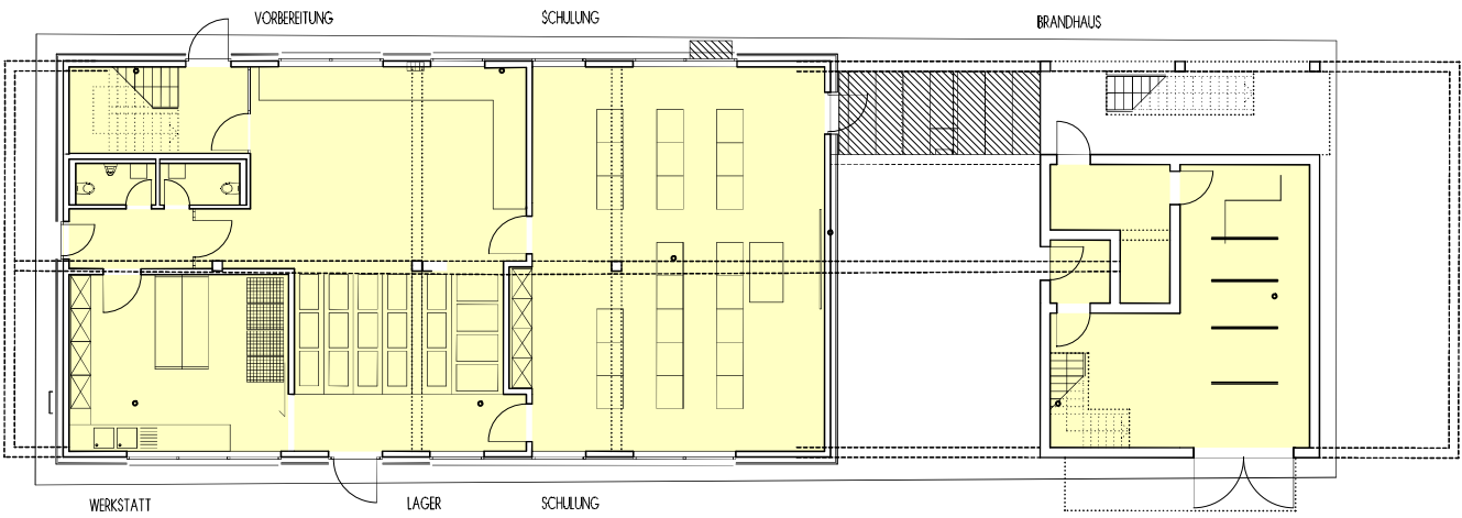
GRUNDRISS EBENE 0
