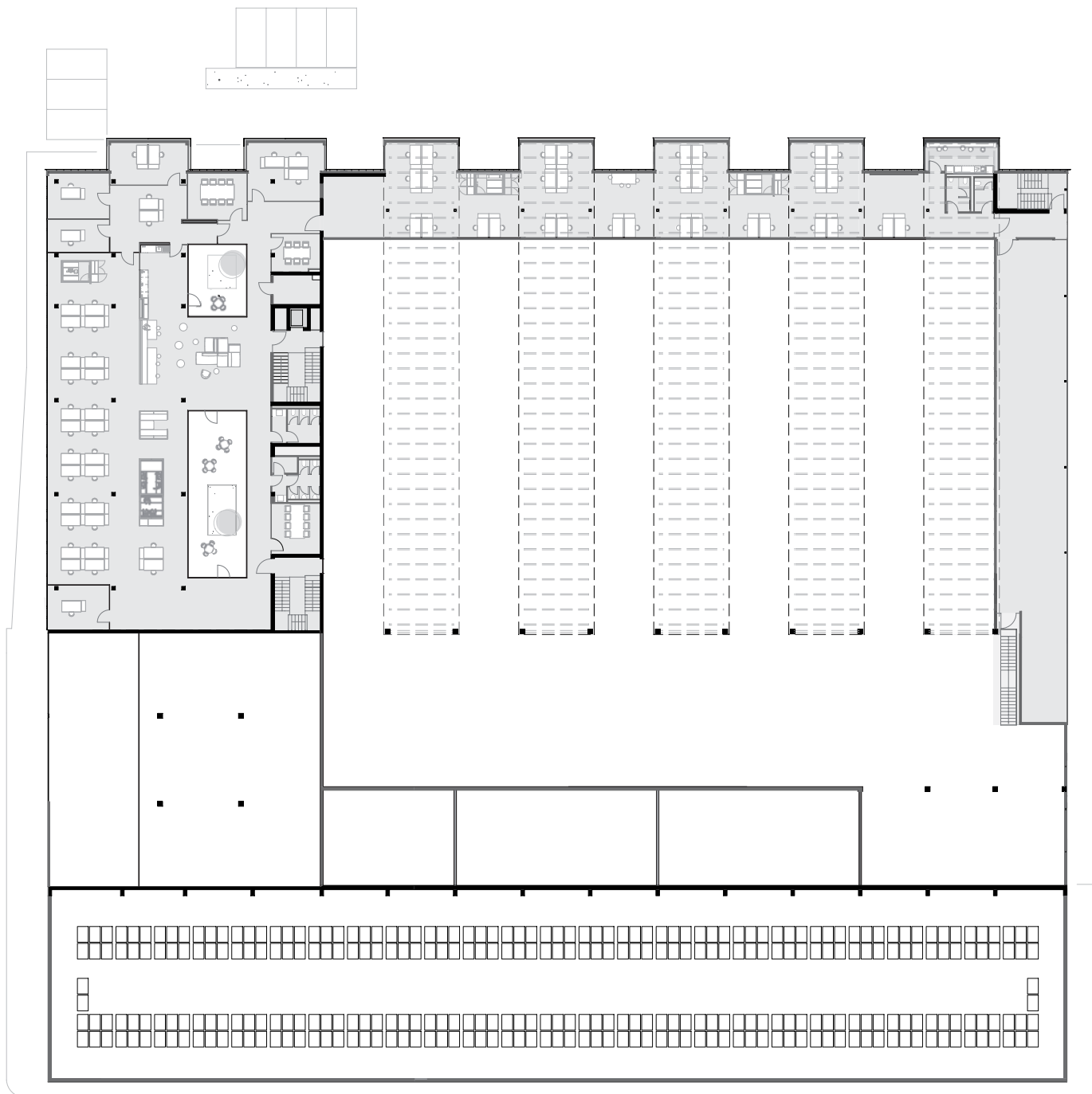
Grundriss 1. OG Headquarter Chemoform Wendlingen a. N.
