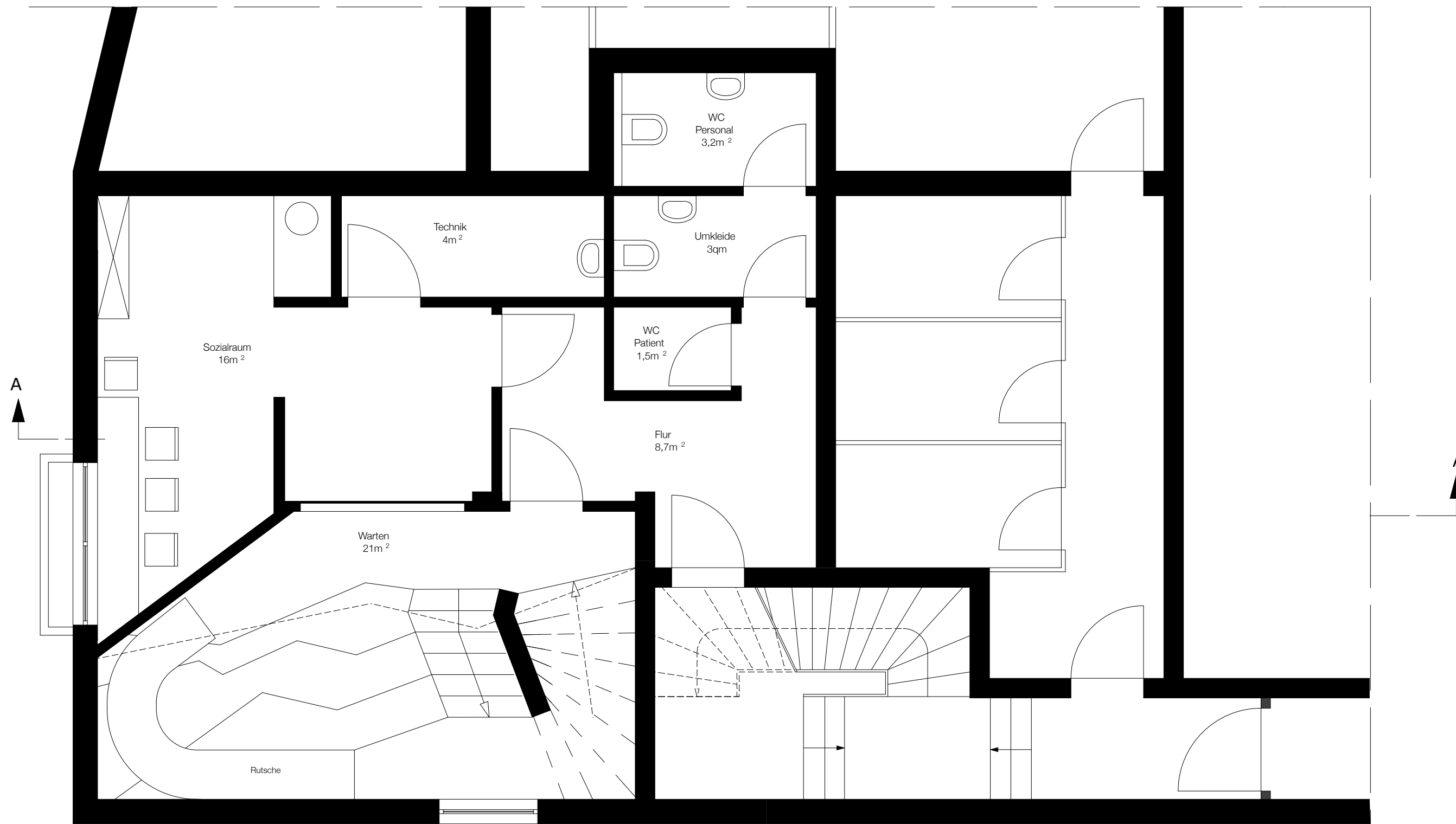
GRUNDRISS UG
