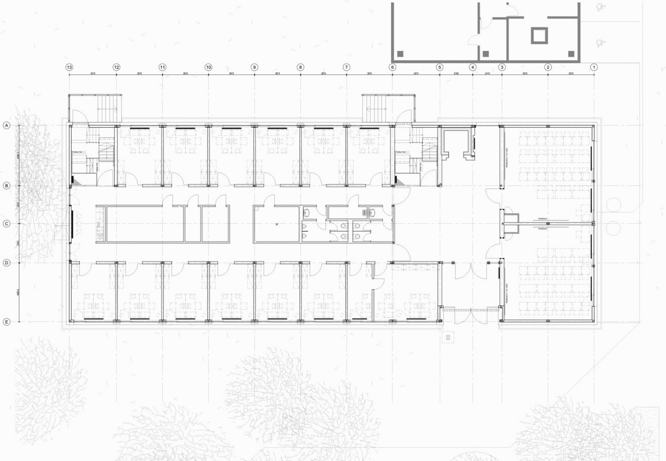
Grundriss EG
