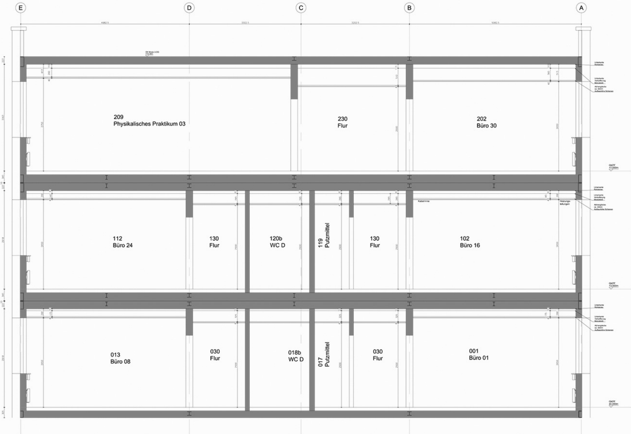
Schnitt
