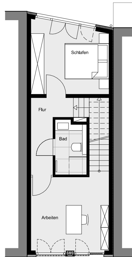
4.Obergeschoss
