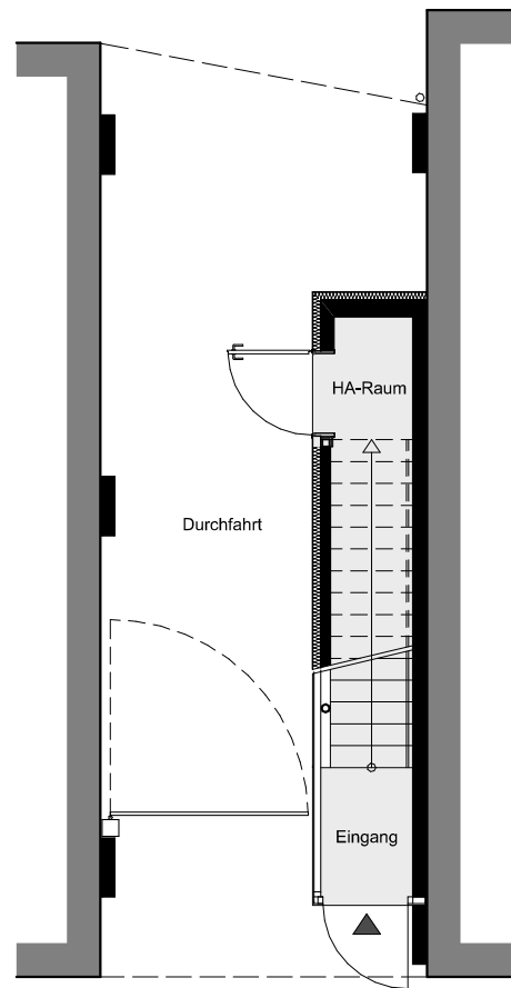
Erdgeschoss
