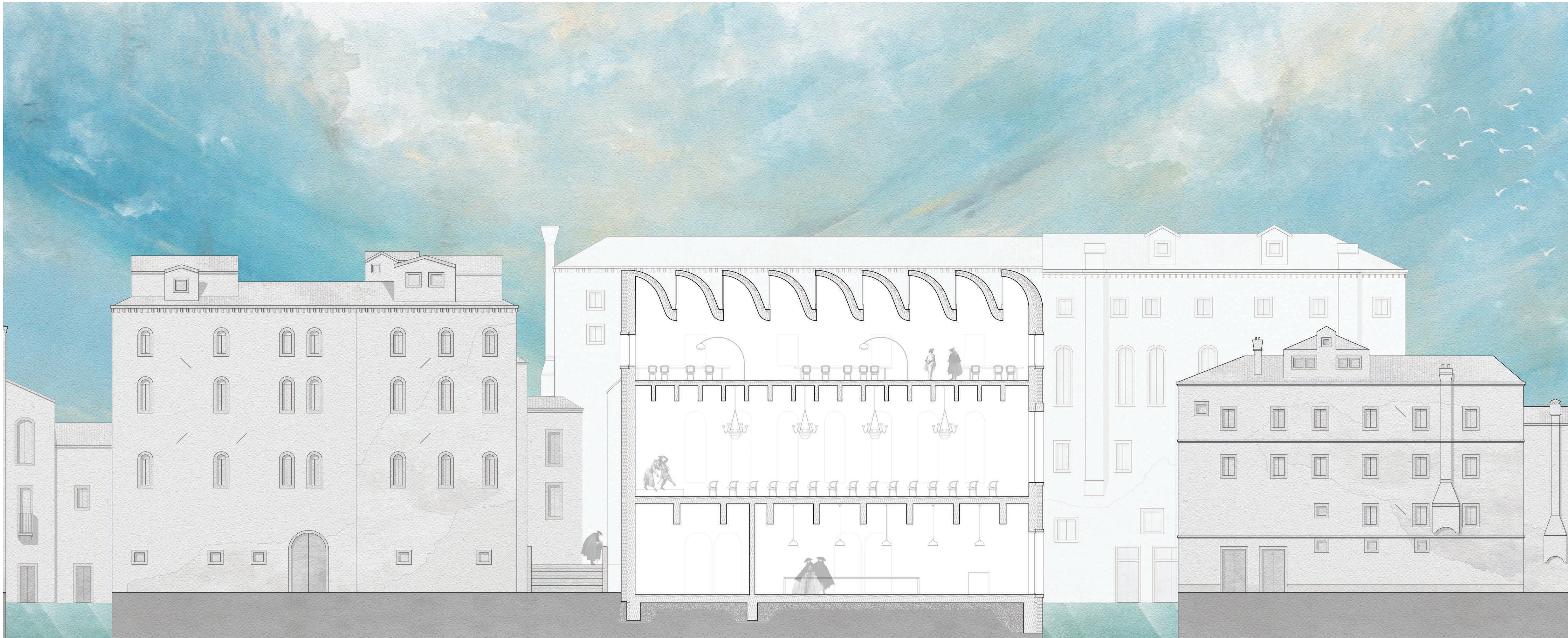
SCHNITT 1:100
