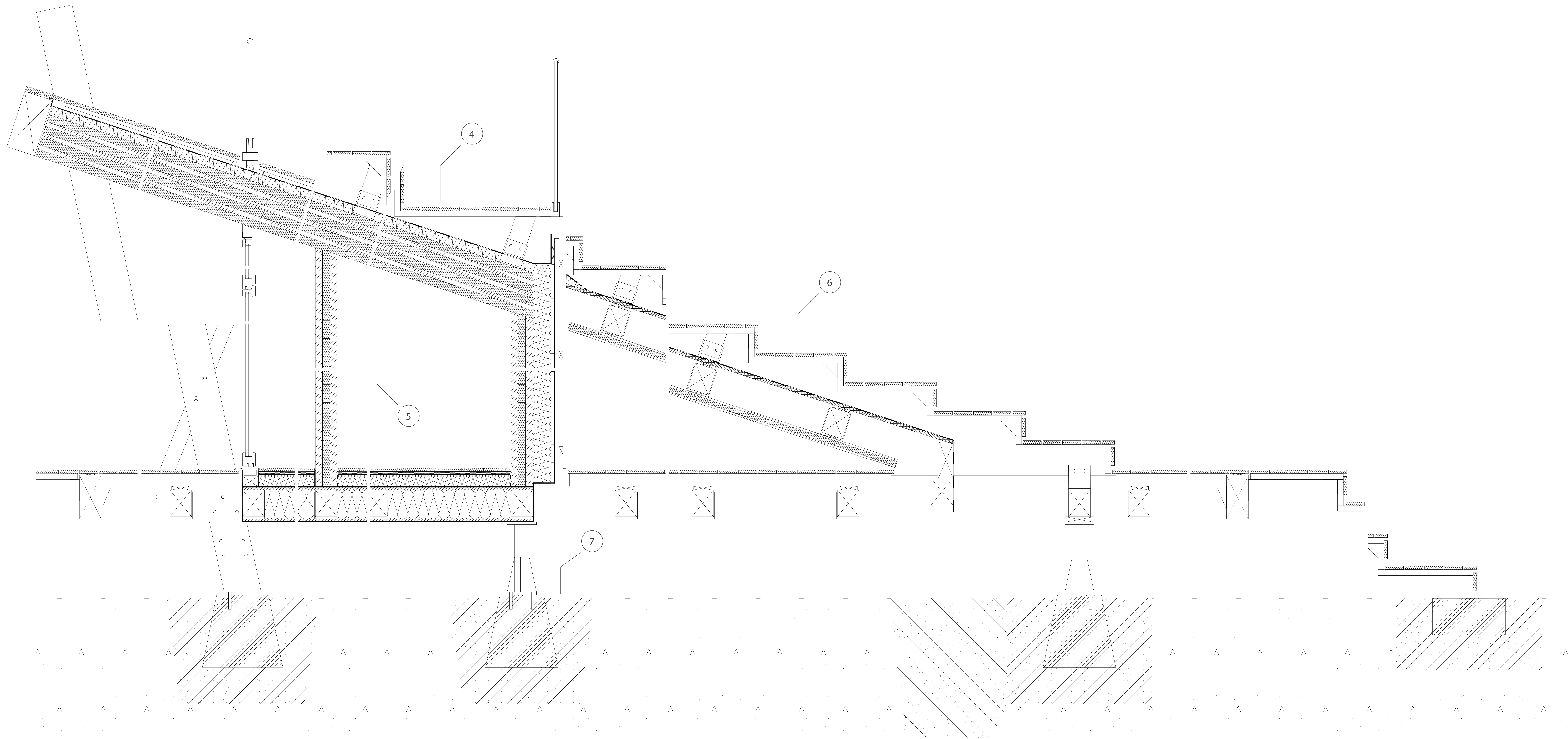
Detailschnitt - Nord-Süd
