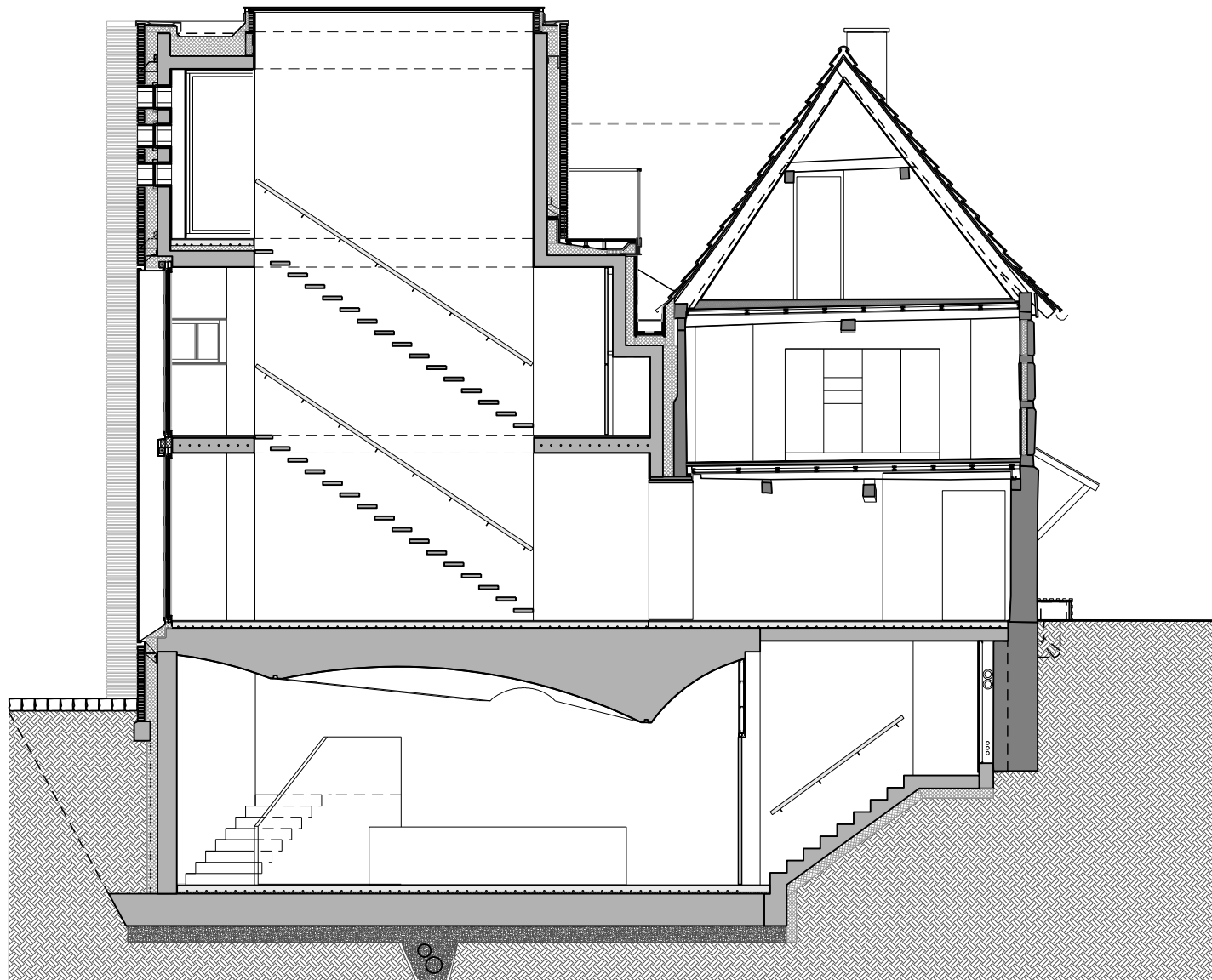
Querschnitt
