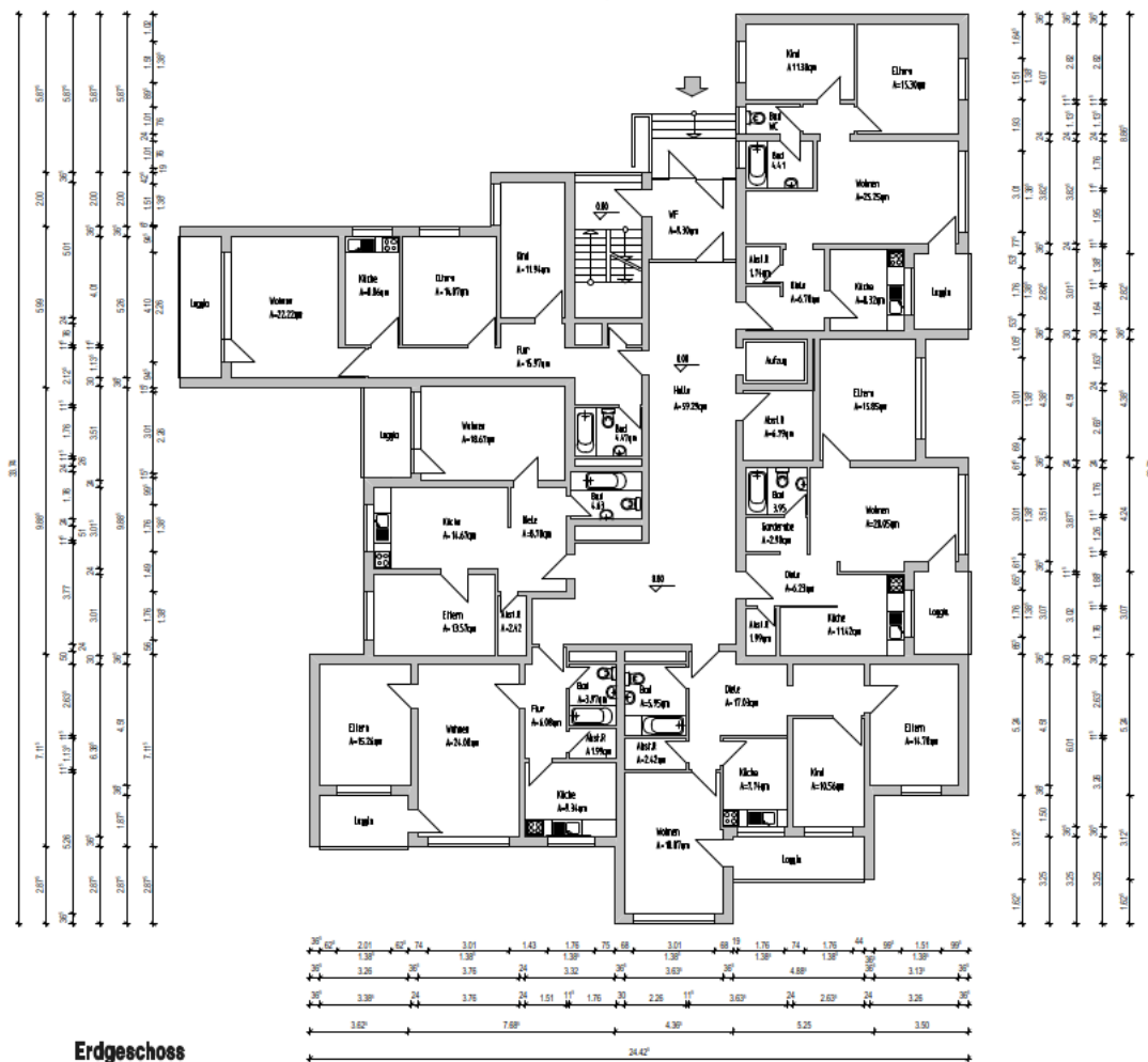
Abbildung 1-1 Grundriss Erdgeschoss
