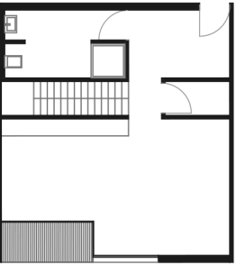
ERDGESCHOSS
