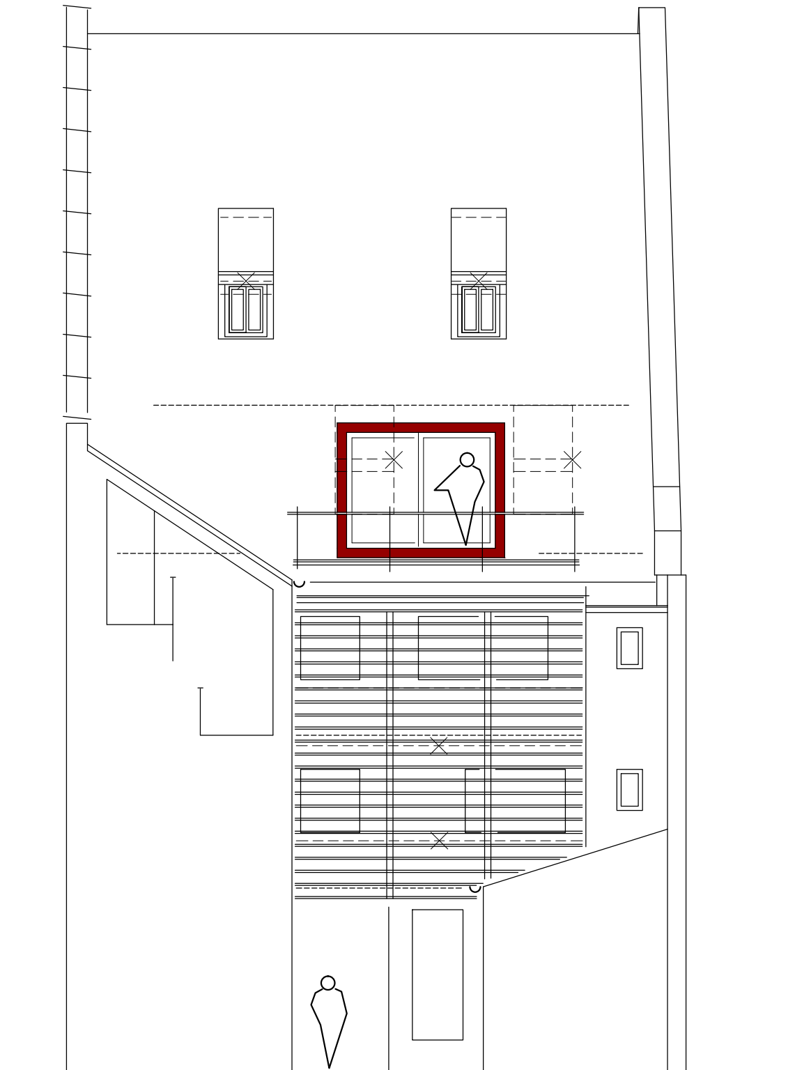
ANSICHT HOFSEITE
