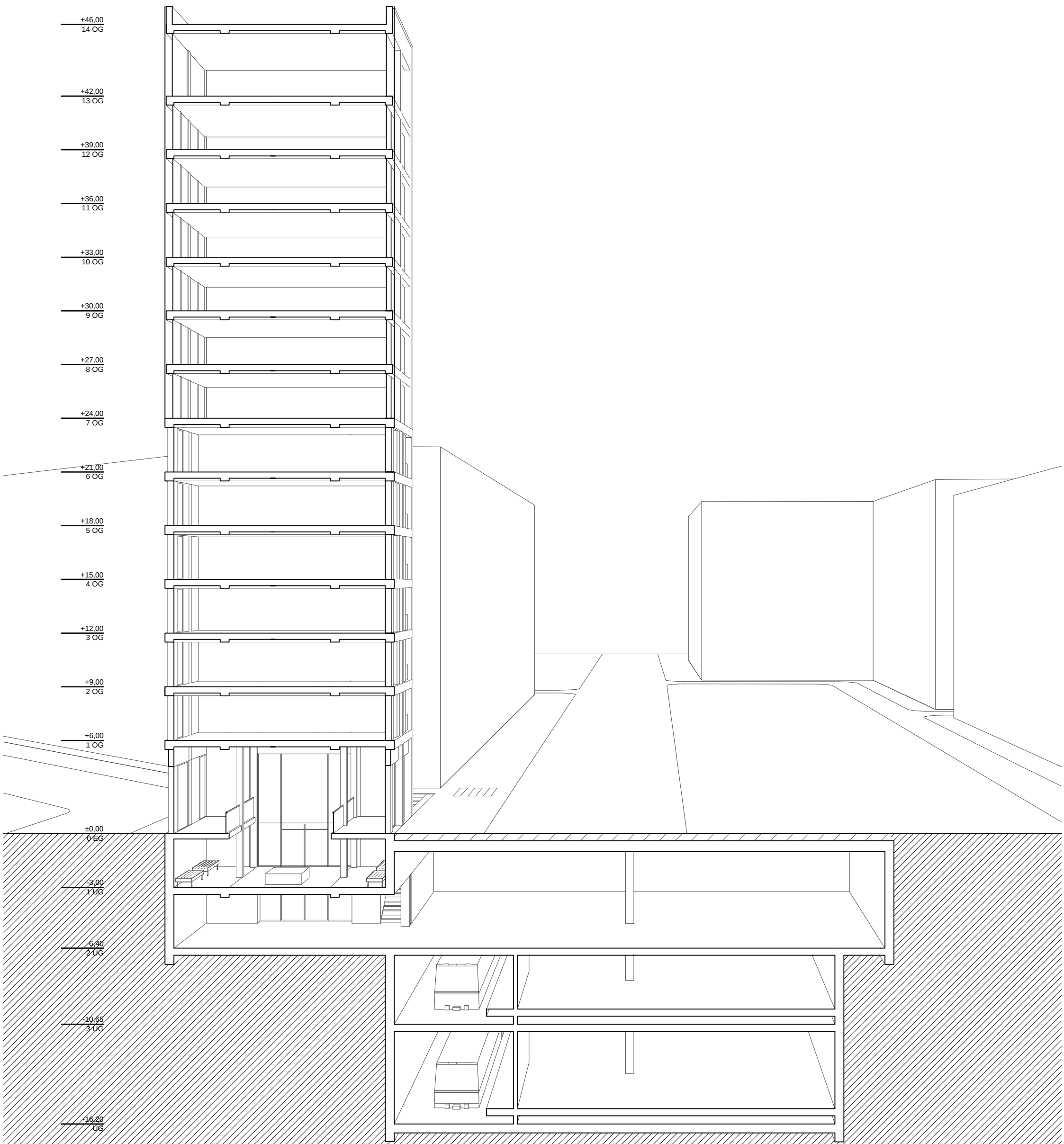
SCHNITT_M1.200
