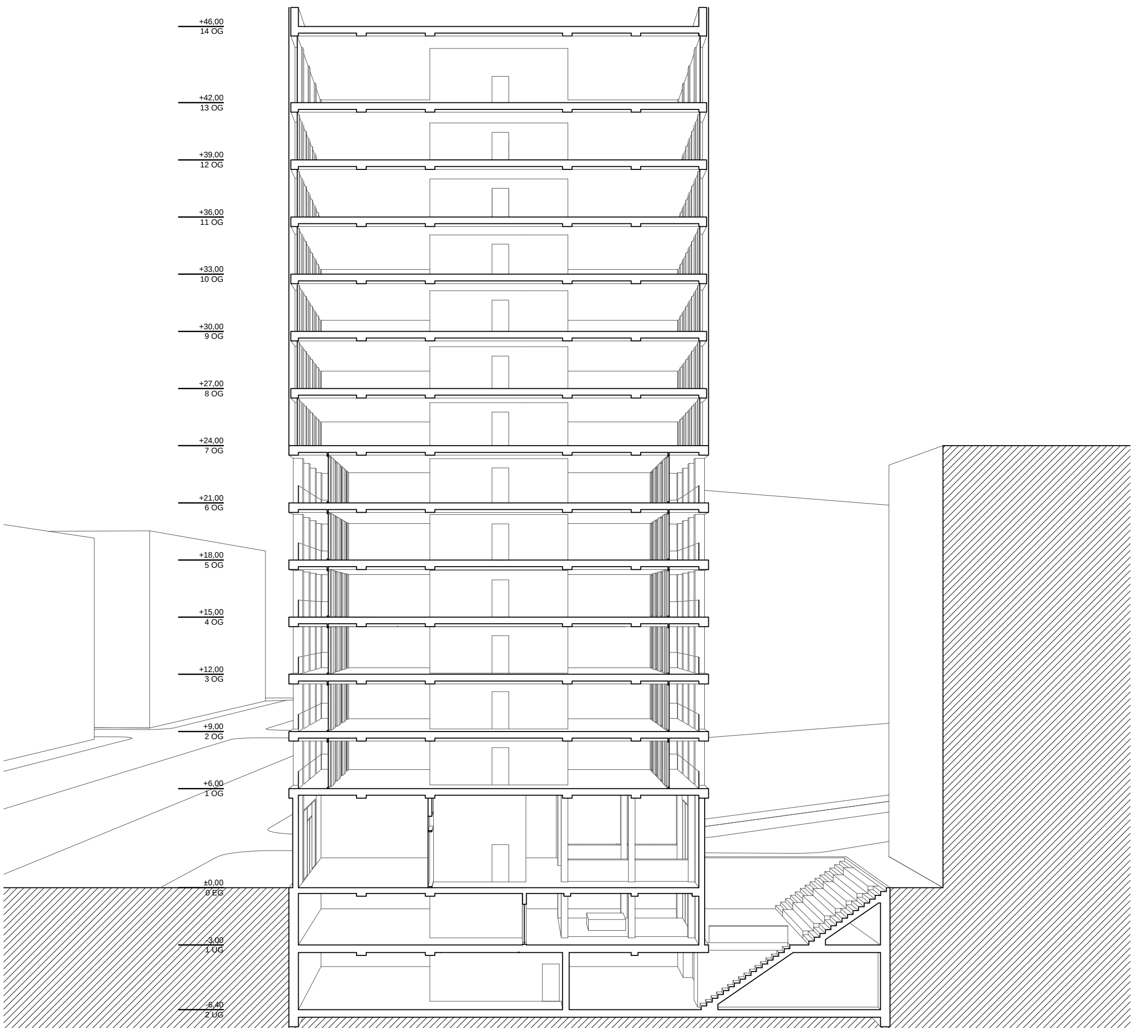
SCHNITT_M1:200
