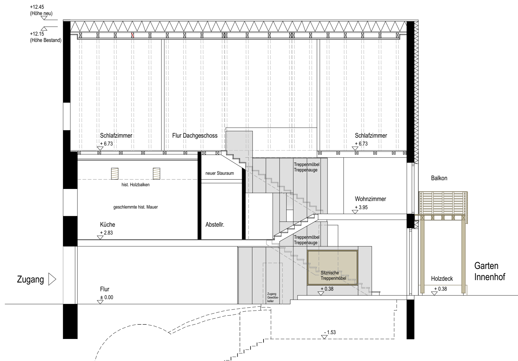
Längsschnitt M 1/100
