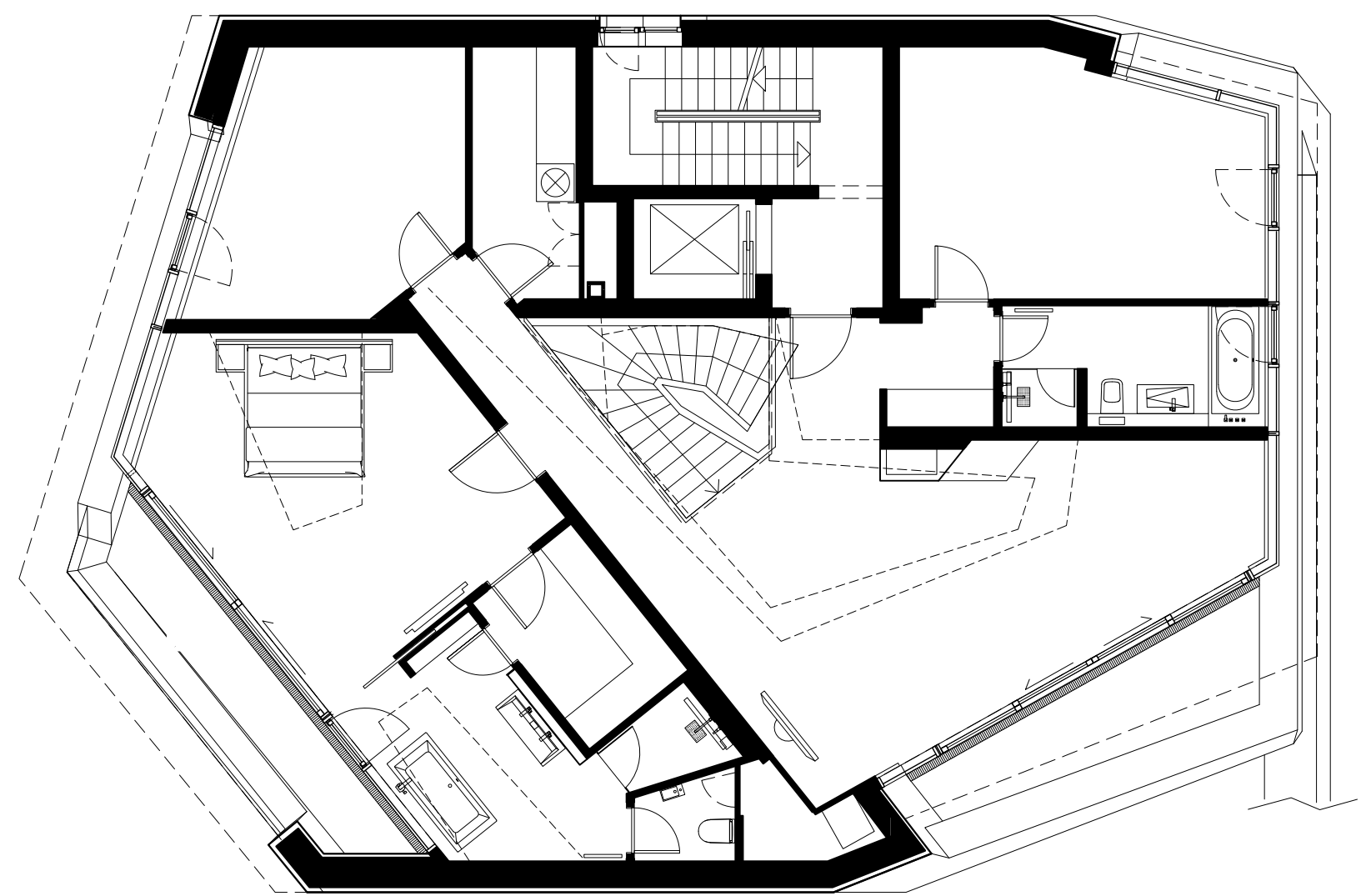
VILLA M OBERGESCHOSS / UPPER LEVEL
