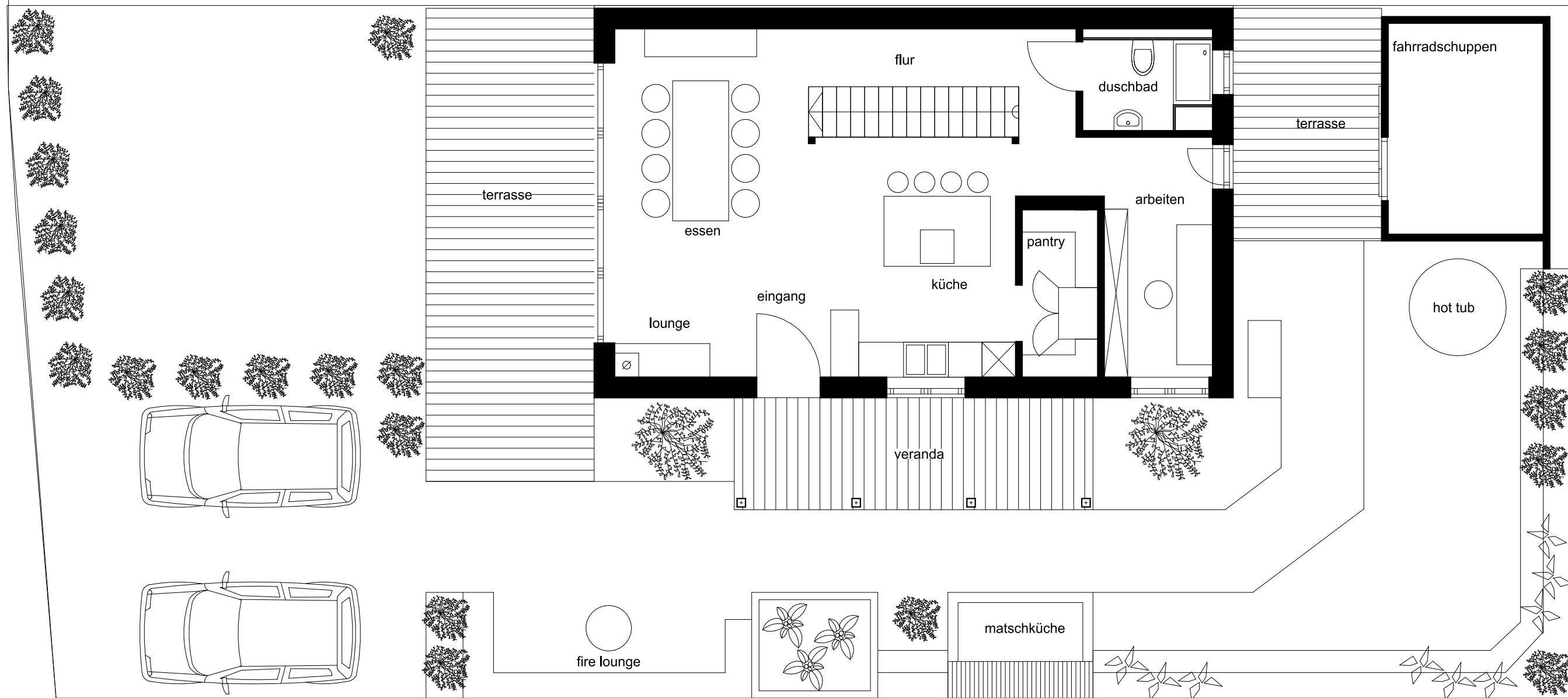
grundriss erdgeschoss
