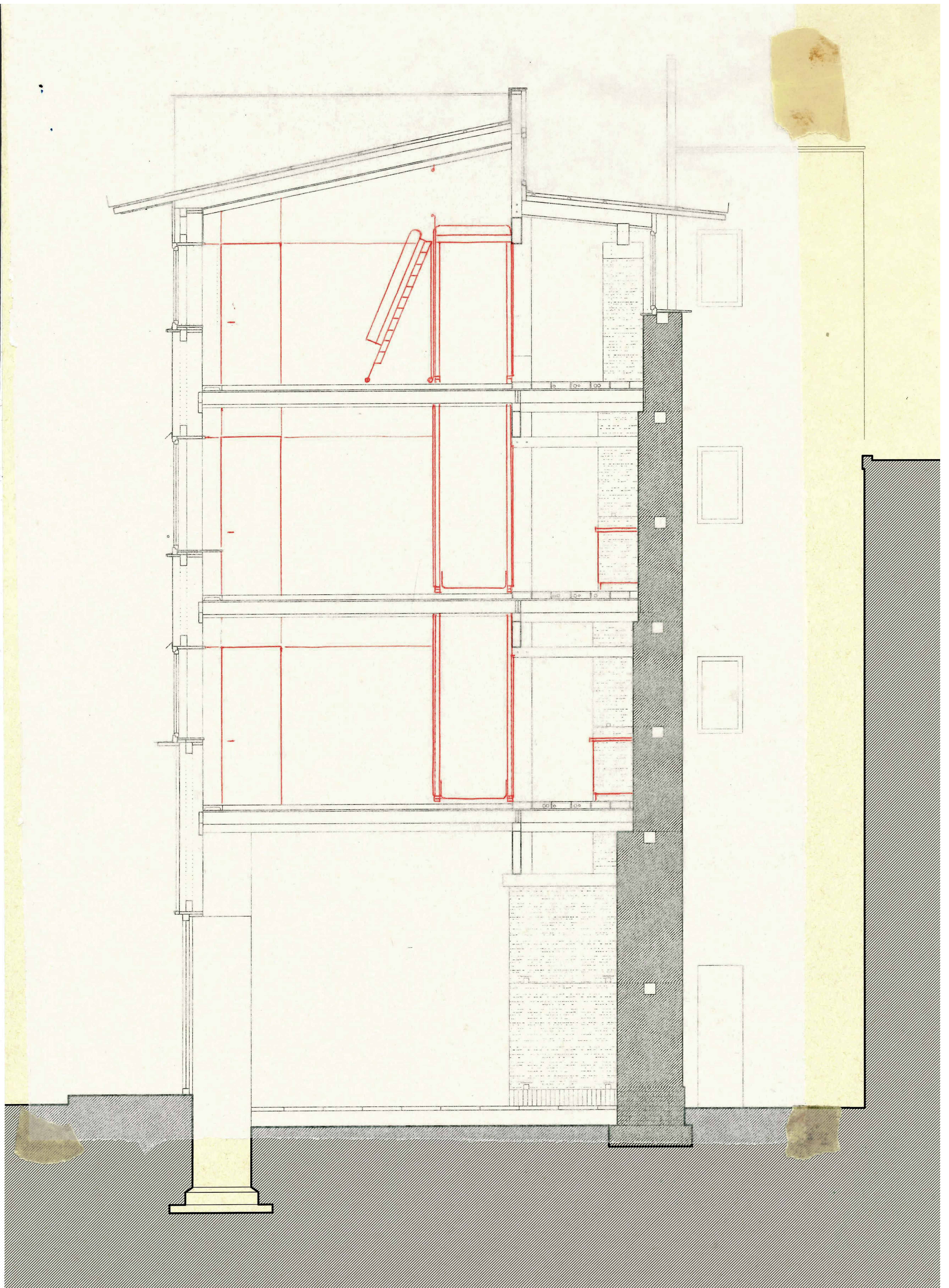
Schnitt,M 1:50
