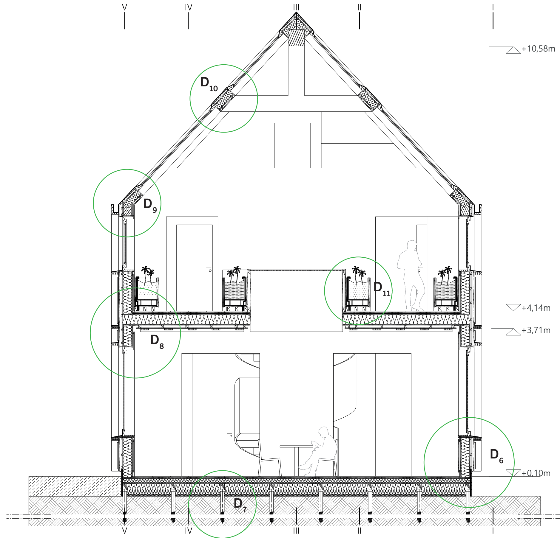
Schnitt F-F M 1:50 (verkleinert)
