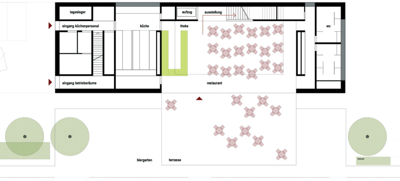
erdgeschoss 1/100
