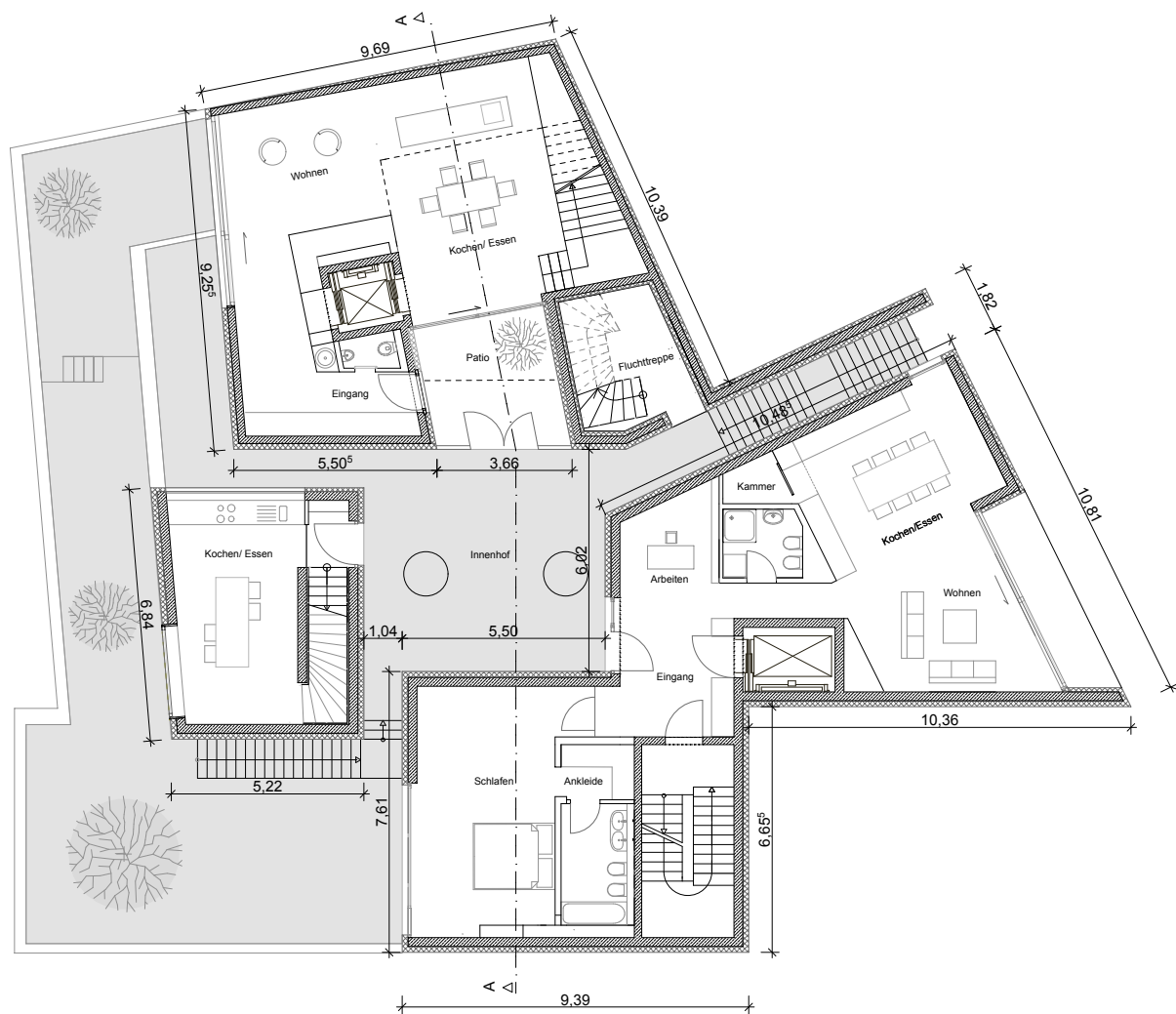
1.OBERGESCHOSS M 1: 200
