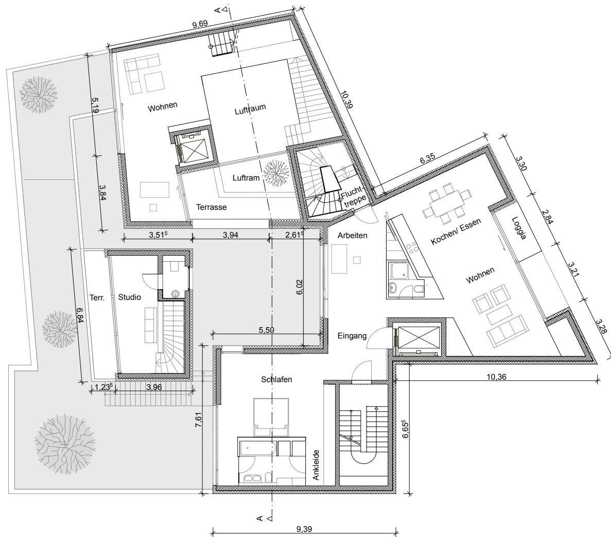
2.OBERGESCHOSS M 1: 200
