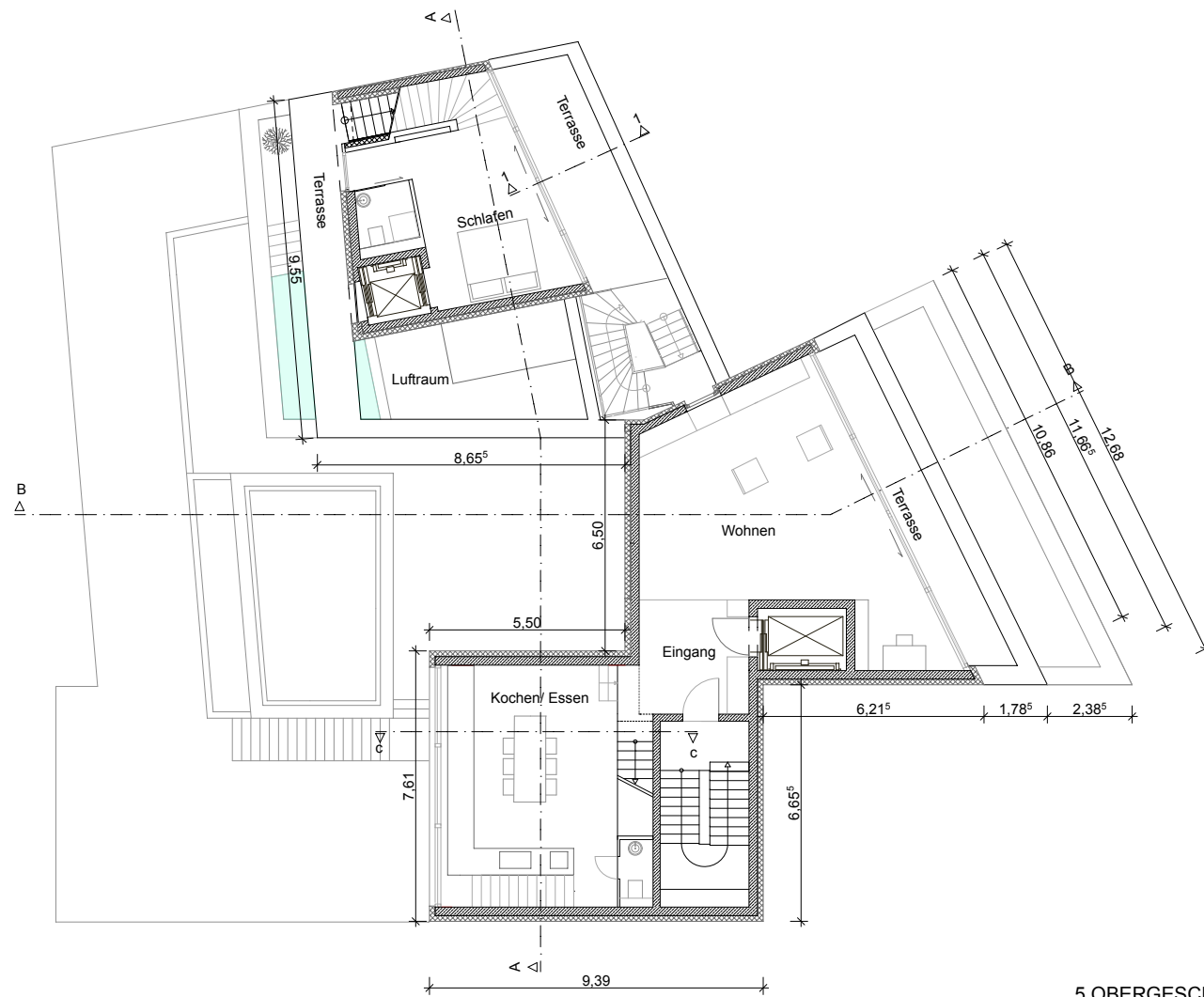
5.OBERGESCHOSS M 1: 200
