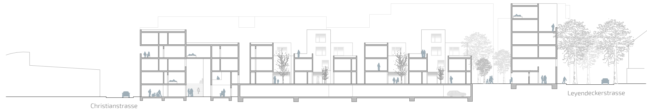
Schnitt B-B M 1:500
