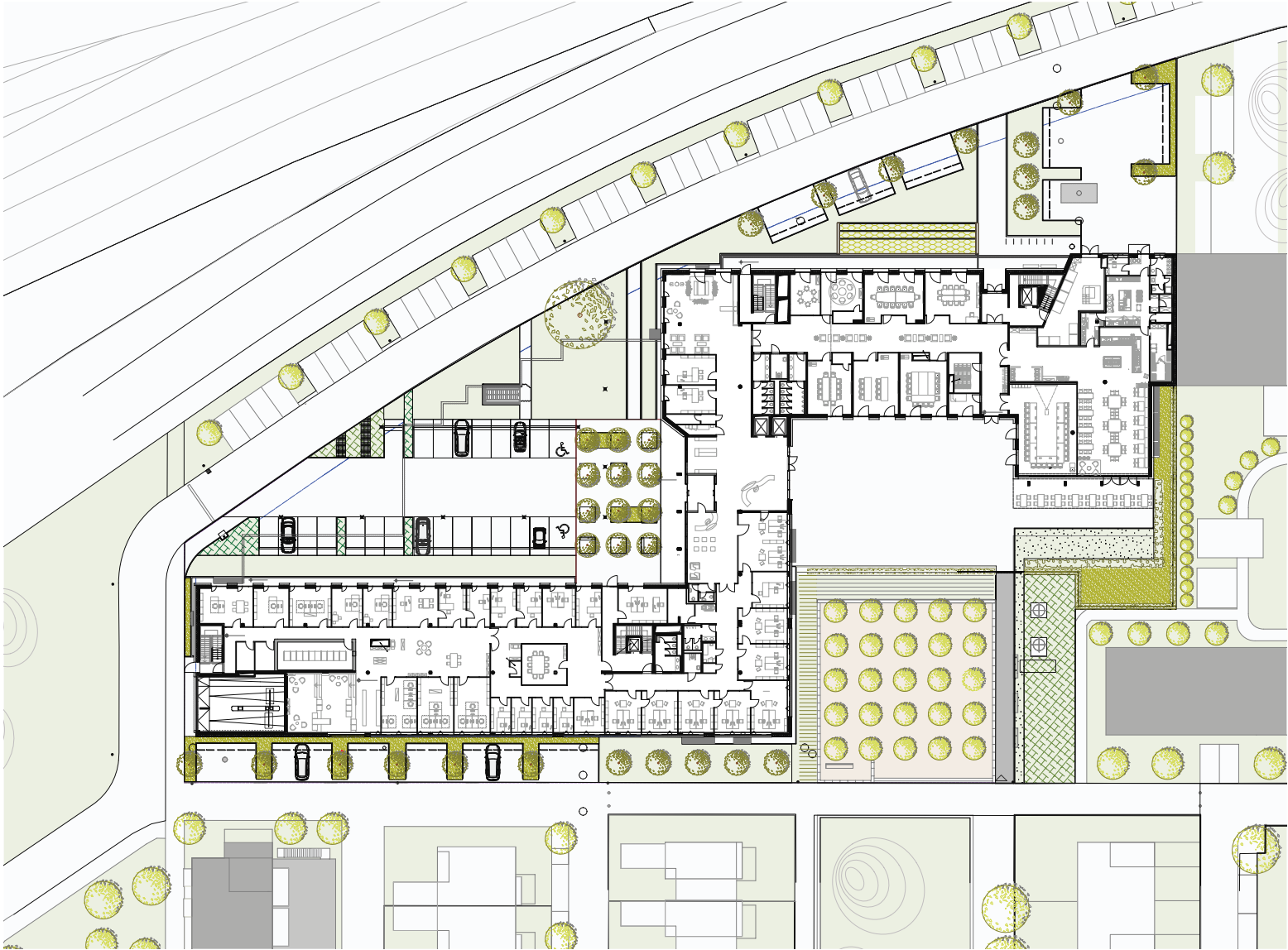
Grundriss Erdgeschoss
