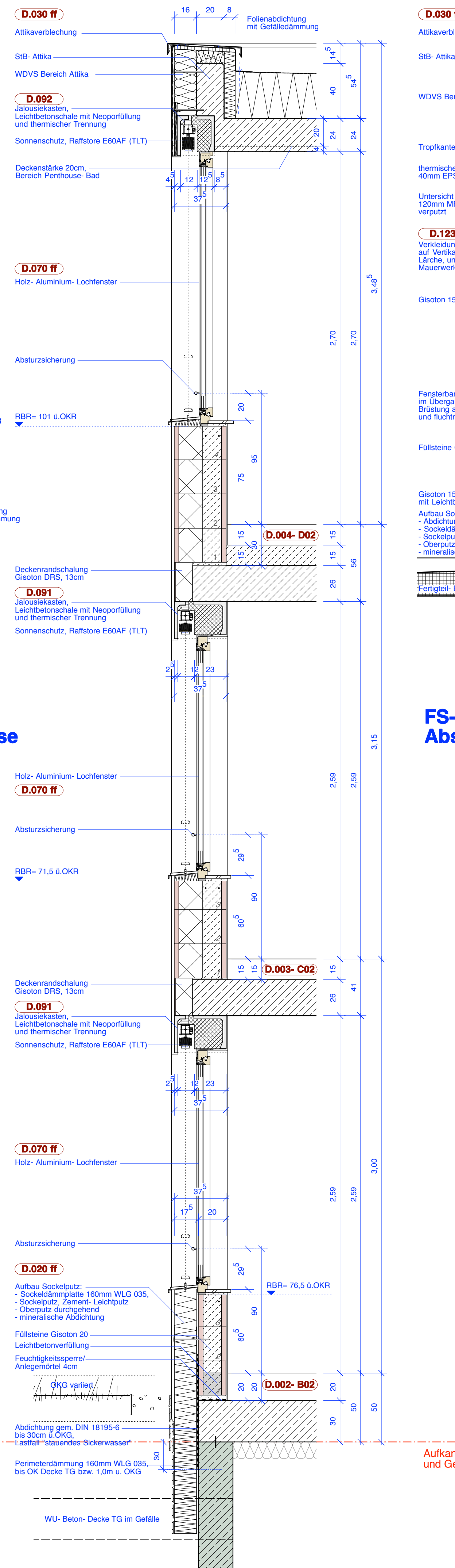
FS-001-B Regelschnitt Lochfenster
