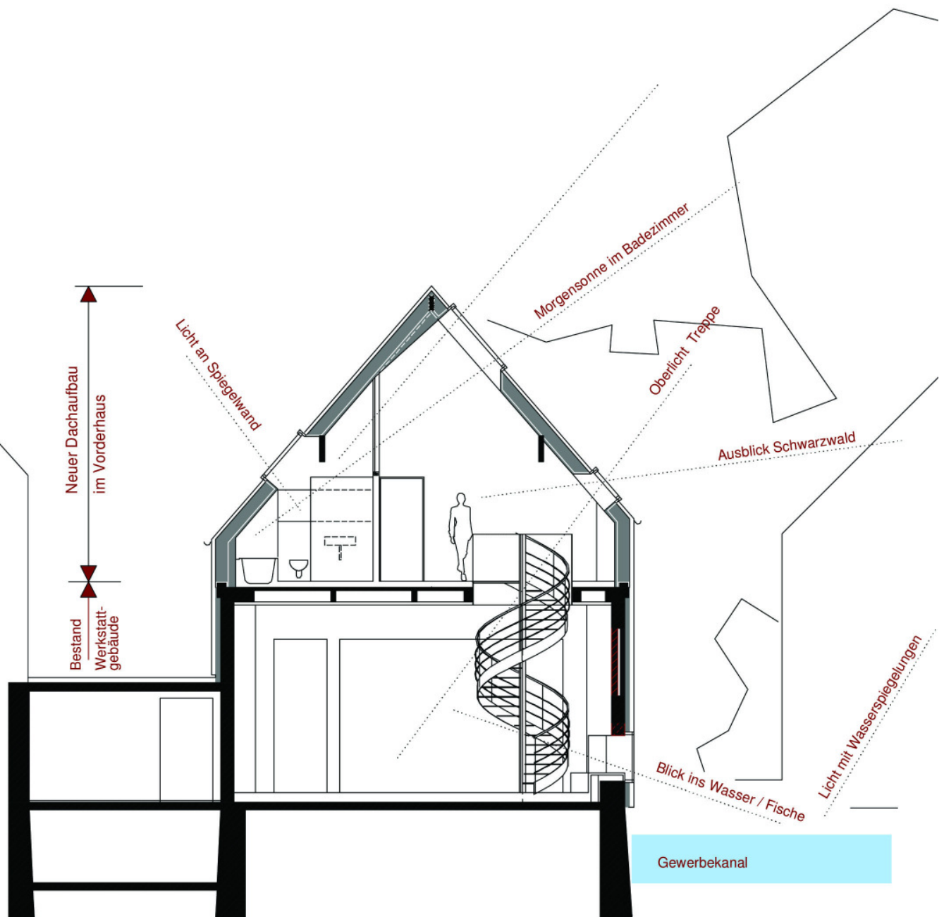
Querschnitt Vorderhaus M: 1:100
