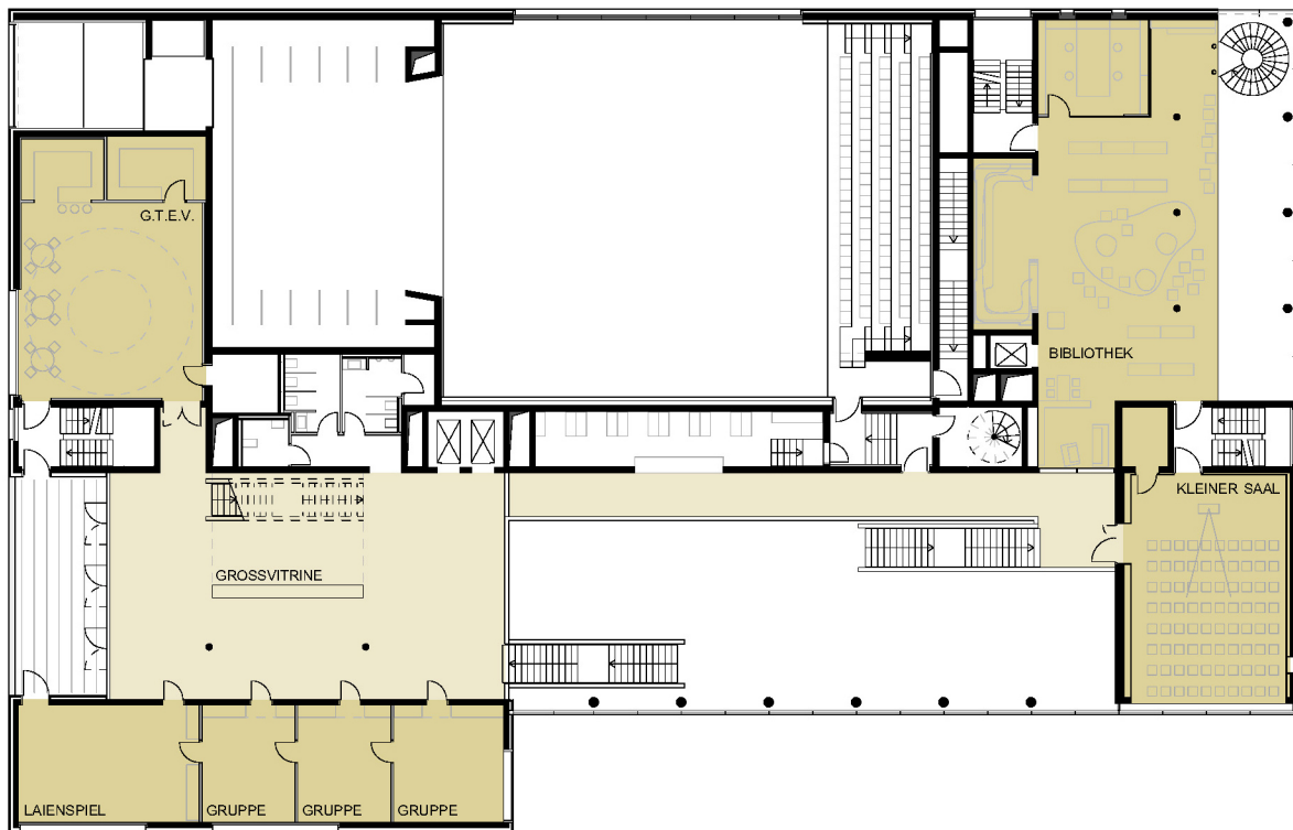
GRUNDRISS 1. OBERGESCHOSS M 1:400
