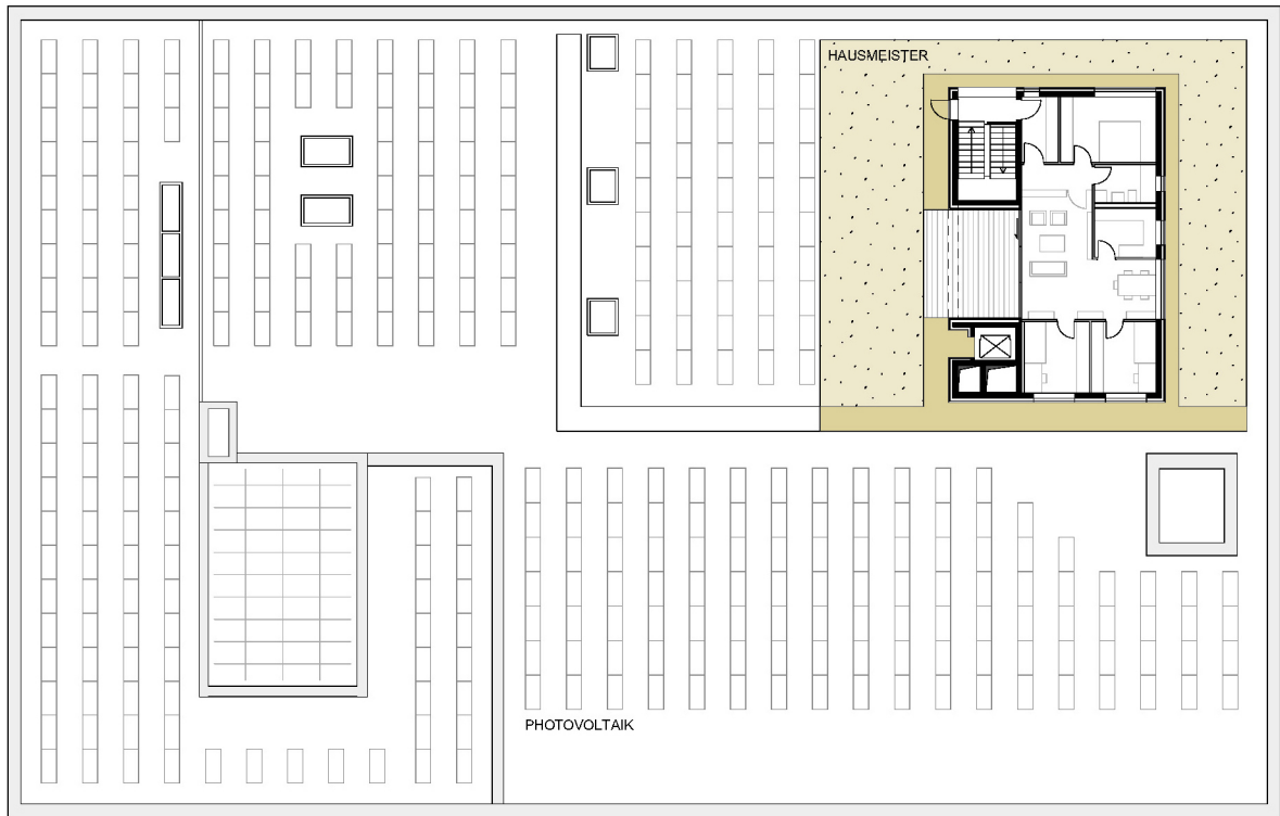
GRUNDRISS 3. OBERGESCHOSS / DACHAUFSICHT M 1:400
