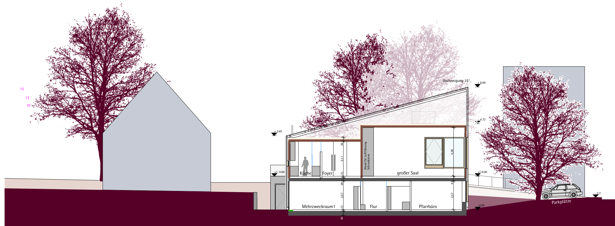
Schnitt A-A
