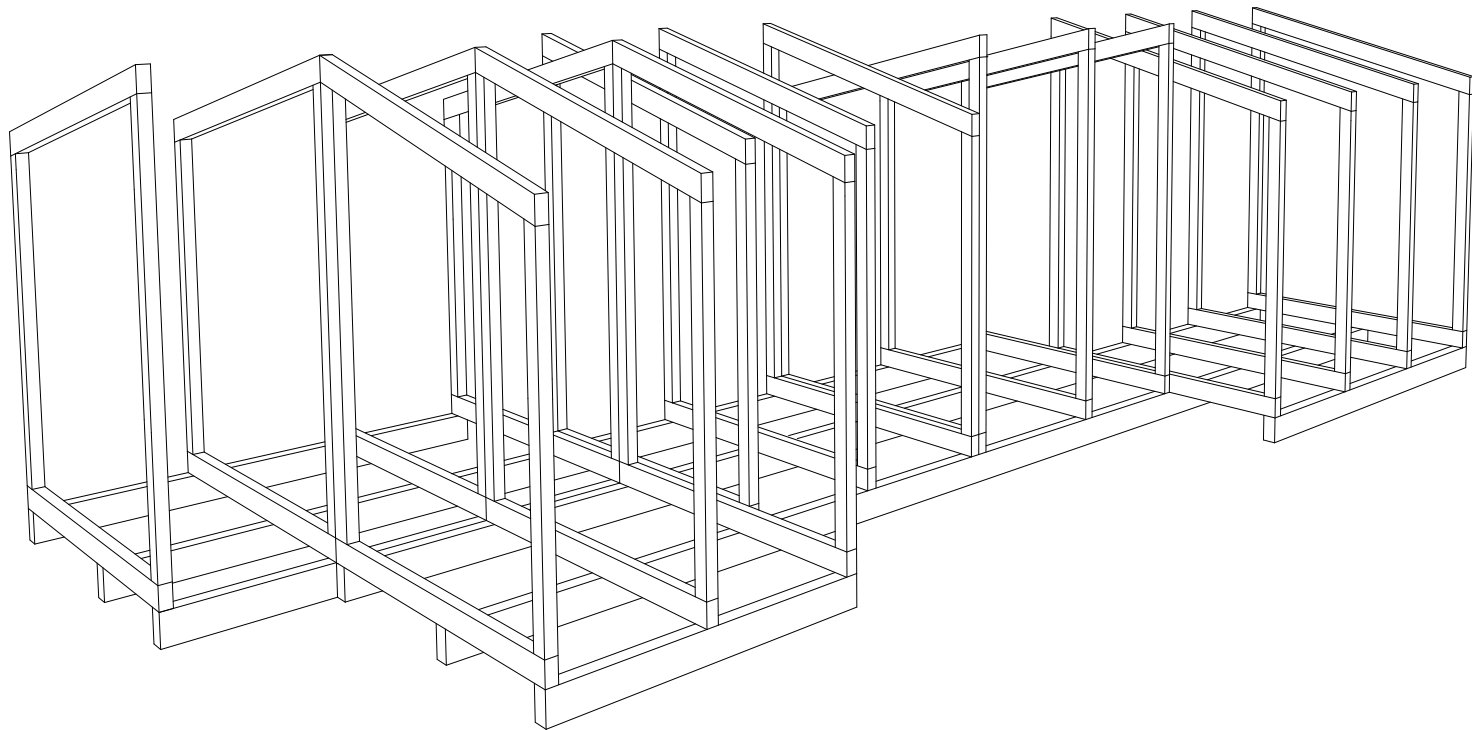
Perspektive Positionierung Modulrahmen
